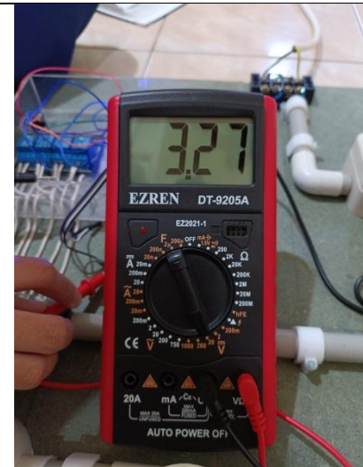
Gambar 8 Tegangan pada IN 2
