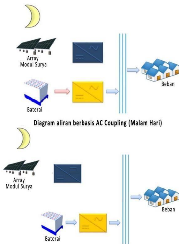
Gambar 2 8 Diagram Aliran Energi pada Malam Hari
