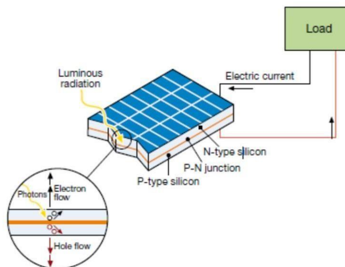
Gambar 2 2Prinsip Kerja Sel Surya
