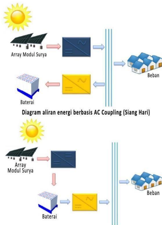
Gambar 2 6 Diagram Aliran Energi yang dihasilkan pada Siang Hari
