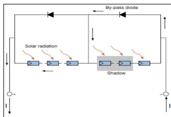
Gambar 2.18 Pengaruh Shading terhadap Modul Surya
