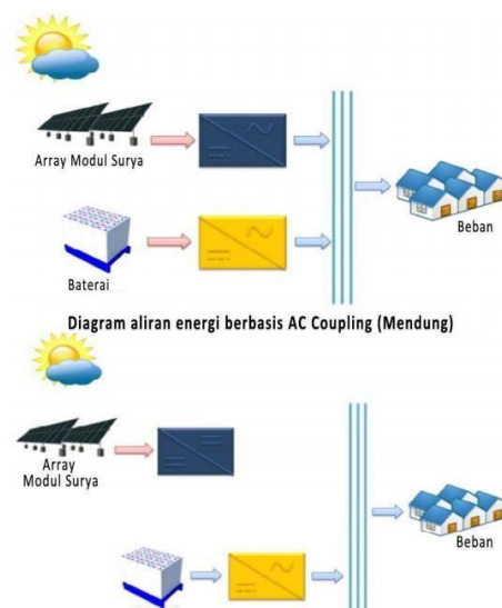
Gambar 2.7 Diagram Aliran Energi yang dihasilkan pada Kondisi Berawan/Mendung
