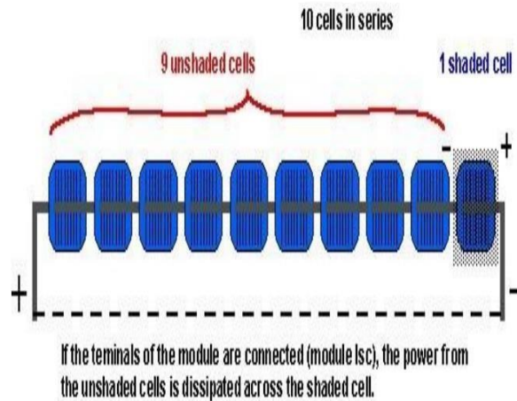
Gambar 2.19 Satu Sel Shading dalam Sebuah String
