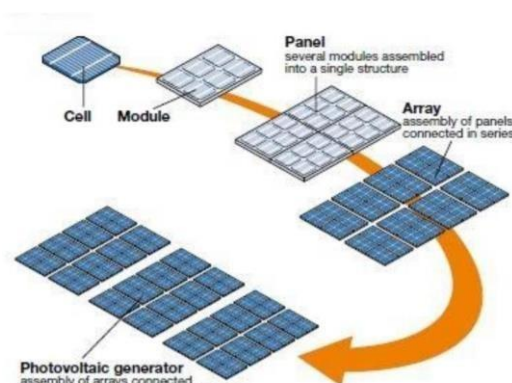
Gambar 2.15 Diagram Hubungan antara Solar Cell, Modul, Panel dan Array
