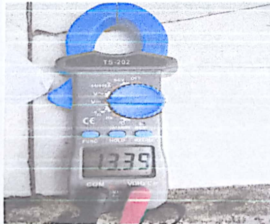
C. Pengambilan Data Tegangan Menggunakan Beban Pompa Air DC
