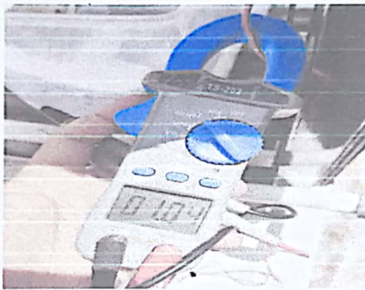
B. Pengambilan Data Arus Pada Pompa Air DC
