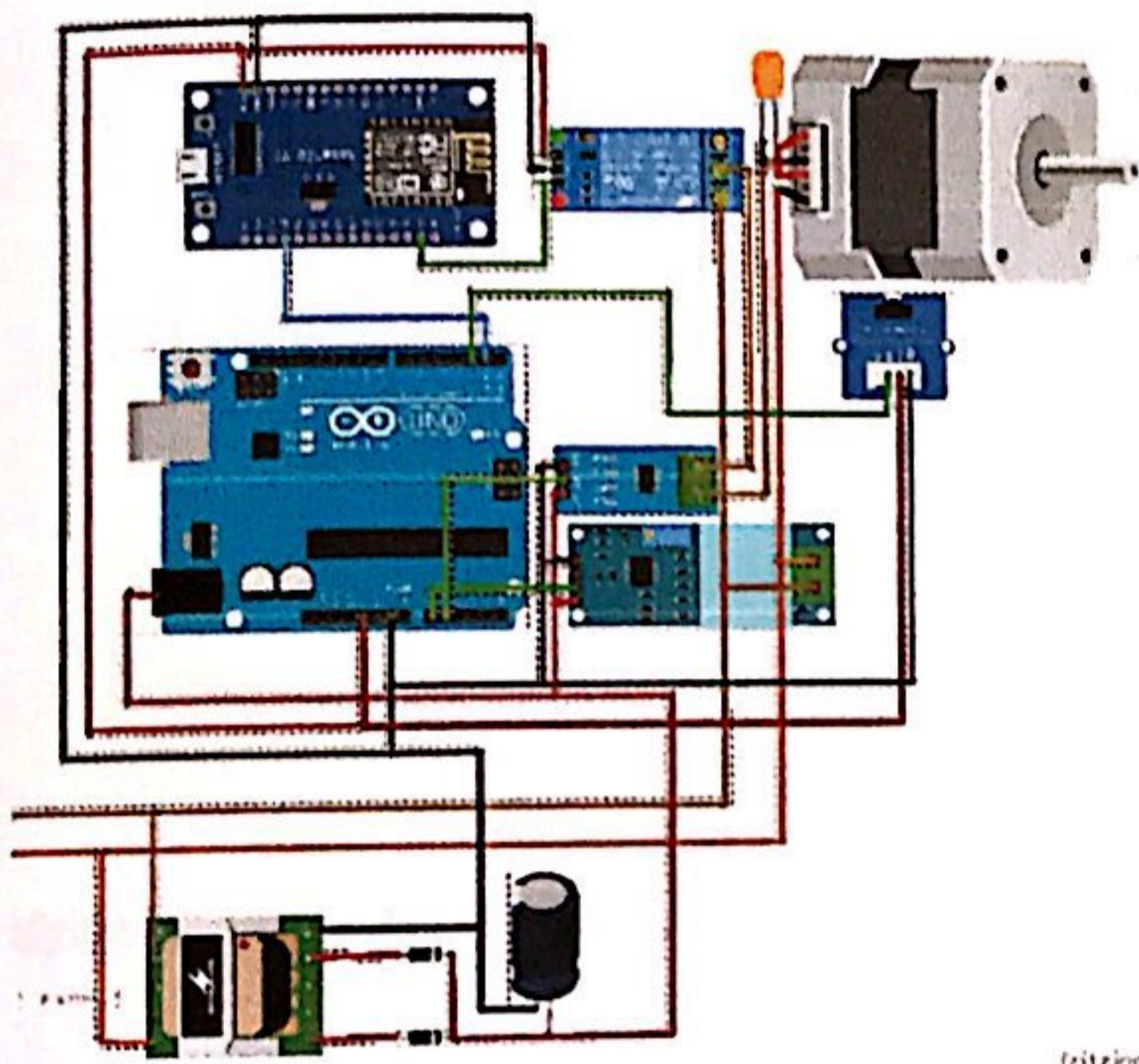
Gambar 2 : Rangkaian Skematik [Sumber : Pribadi]
