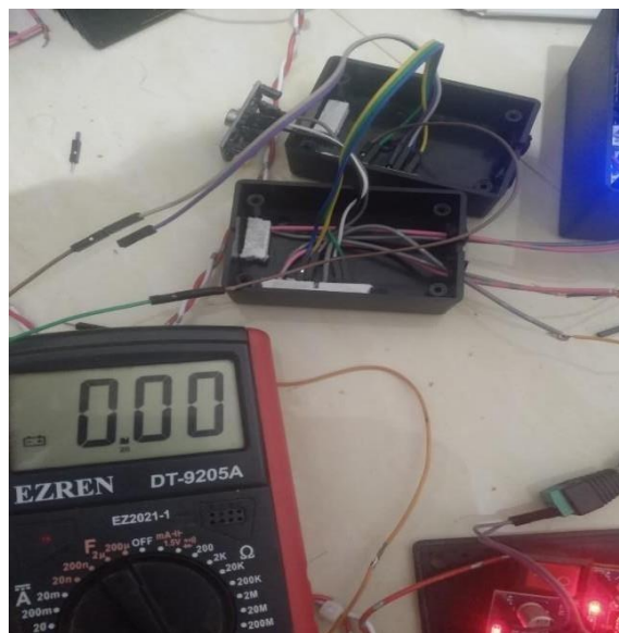
Pengukuran pada output sensor pir
