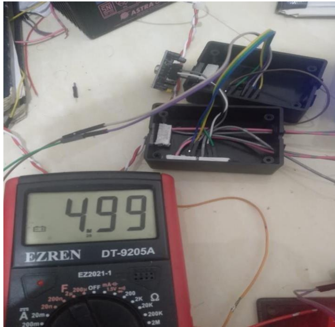
Pengukuran pada input sensor pir
