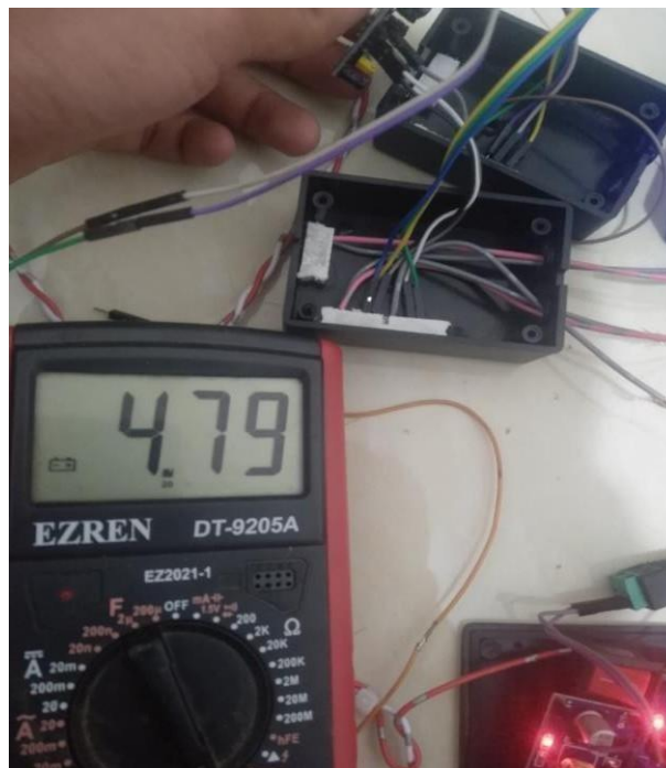
Pengukuran pada input sensor pir
