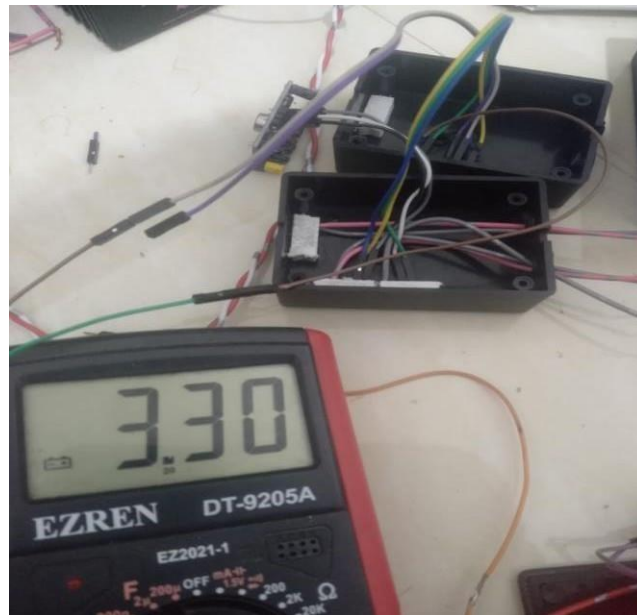
Pengukuran pada output sensor pir
