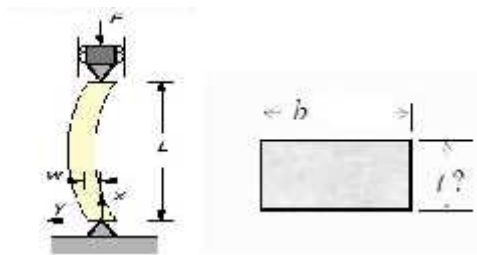
Gambar 2.8 beban bengkok dan tebal pelat
