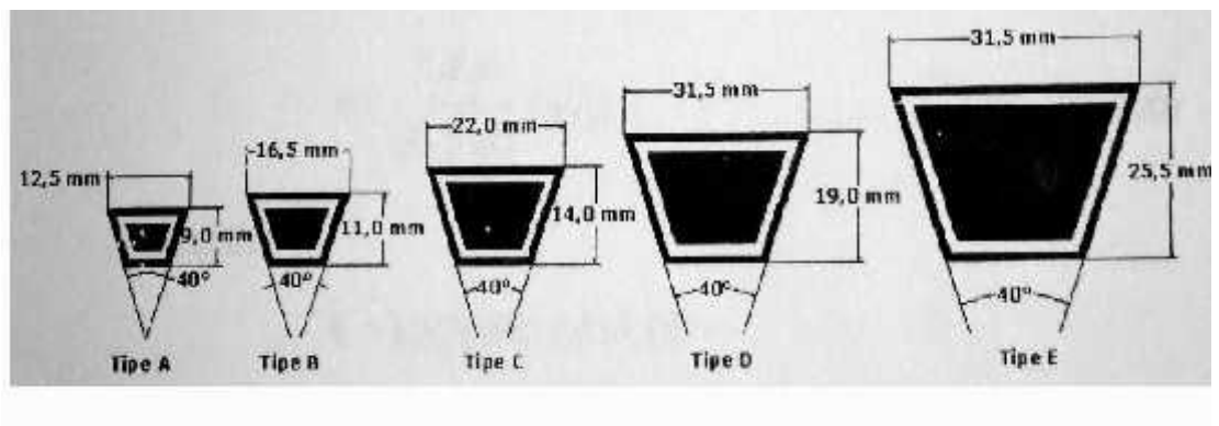
Gambar 2.6 Ukuran penampang sabuk V
