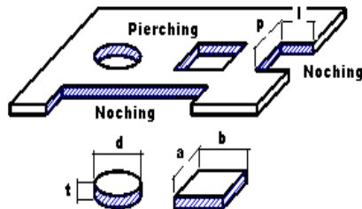
Gambar 2.31 Permukaan pelat yang di Notching dan Pierching
