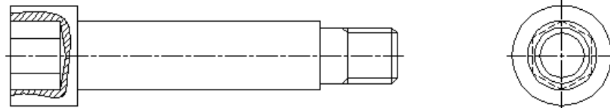
Gambar 2.27 Baut Pemegang
