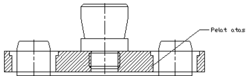
Gambar 2.17 Pelat Atas
