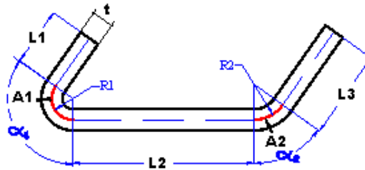
Gambar 2.30 Pelat sudah di bending
