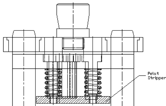
Gambar 2.20 Pelat Stripper
