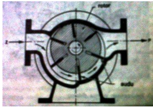
Gambar 2.3 Pompa dinding Sumber: literatur 2
