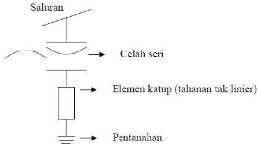
Gambar 2.19 Konstruksi Valve Type Arrester
