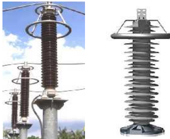
Gambar 2.16 Lightning Arrester di Gardu Induk 12
