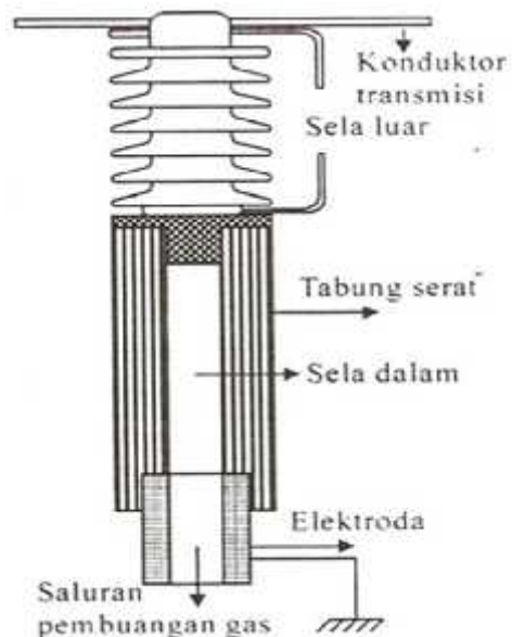
Gambar 2.17 Arrester jenis ekspulsi 13
