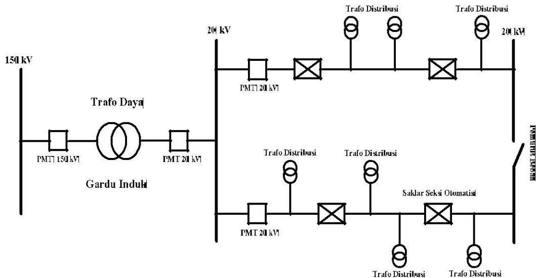
Gambar 2.3 Jaringan Distribusi Sistem Loop
