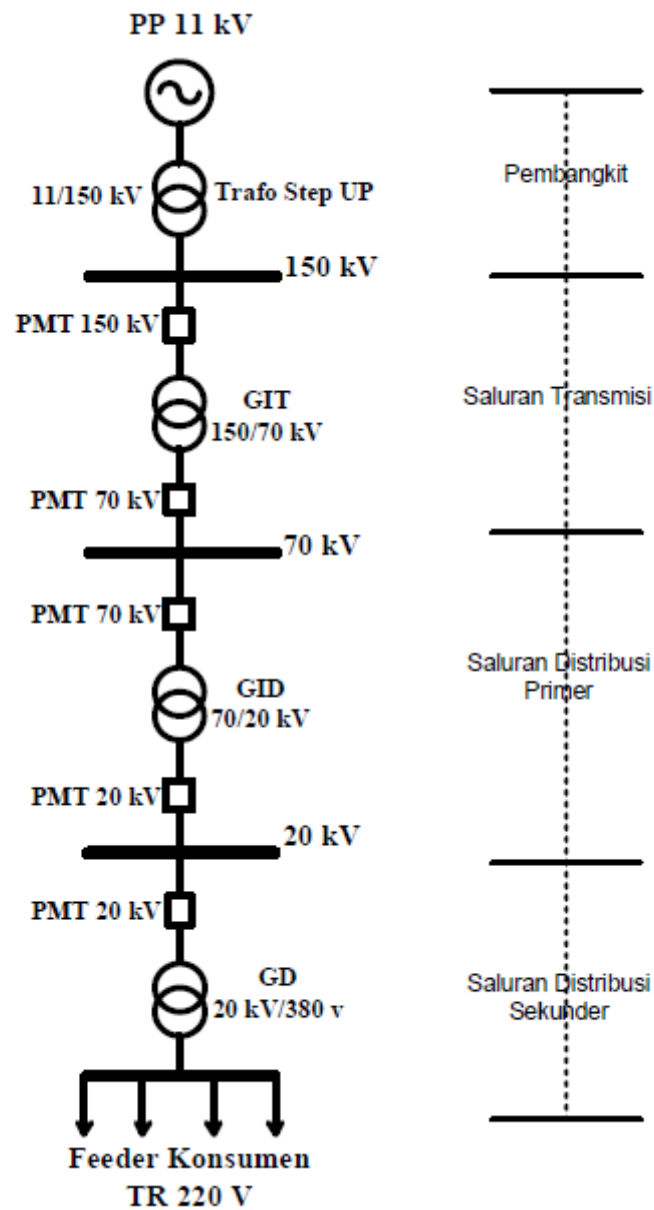
Gambar 2.1 Sistem Tenaga Listrik 2
