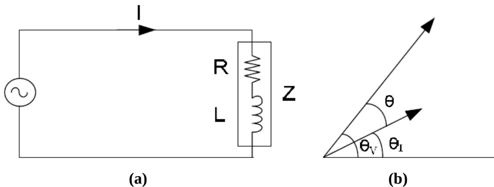
Gambar 2.7 Tegangan AC yang diterapkan pada beban dan diagram fasor.
