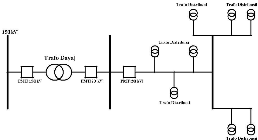
Gambar 2.2 Jaringan Distribusi Sistem Radial
