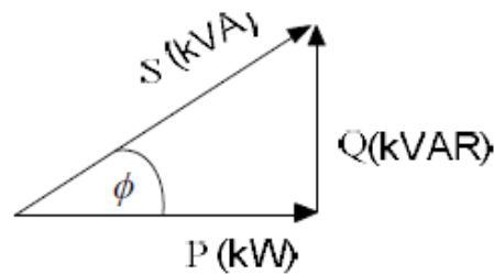
Gambar 2.8 Segitiga Daya Kompleks
