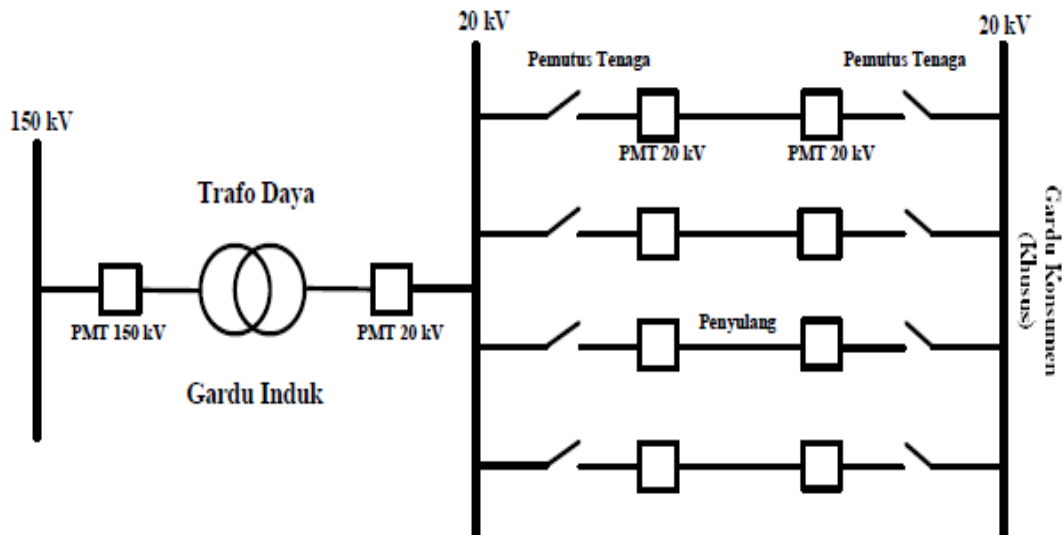
Gambar 2.4 Jaringan Distribusi Sistem Ring
