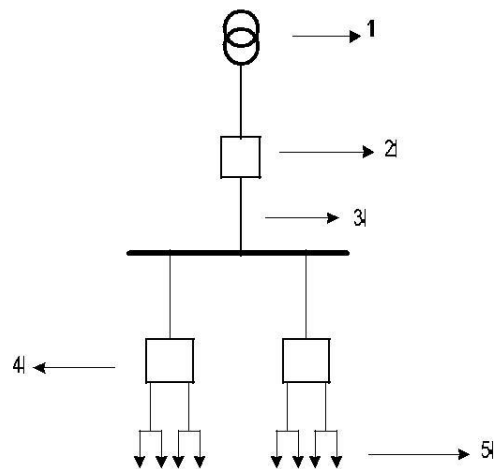
Gambar 2.6 Bagian-Bagian Sistem Distribusi Primer
