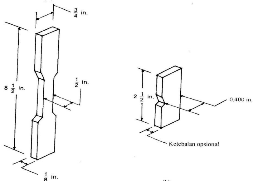
Gambar 1. Spesimen-Spesimen Uji Plastik Khas untuk Mengukur Kekuatan Tensil dan Impak
