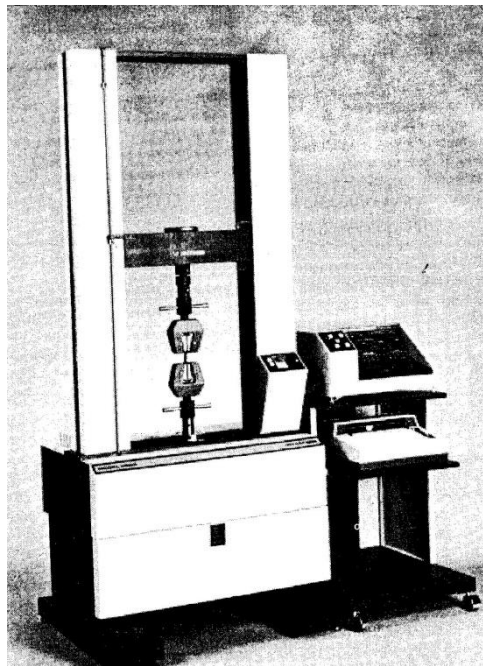
Gambar 2. Instrumen untuk Melakukan Pengujian Tensil, Kompresi, Pengujian Penggungtingan dan Pengujian Kelenturan
