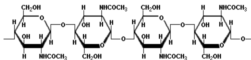
Gambar 6. Struktur Chitin
