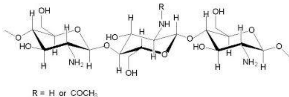
Gambar 7. Struktur Chitosan
