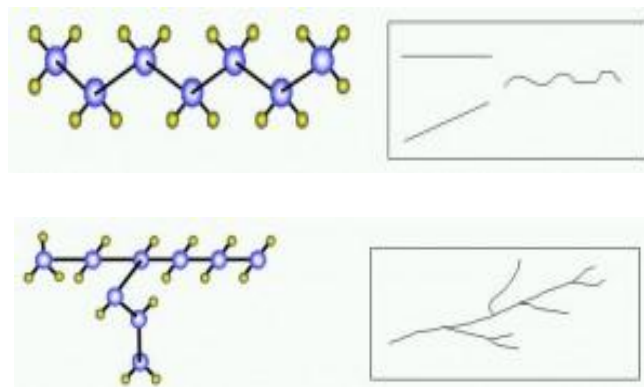
Gambar 3. Bentuk Struktur Bercabang Termoplastik
