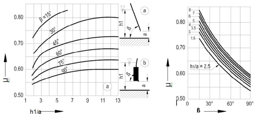
Gambar 2.7 Koefisien debit \mu masuk permukaan pintu datar atau lengkung
