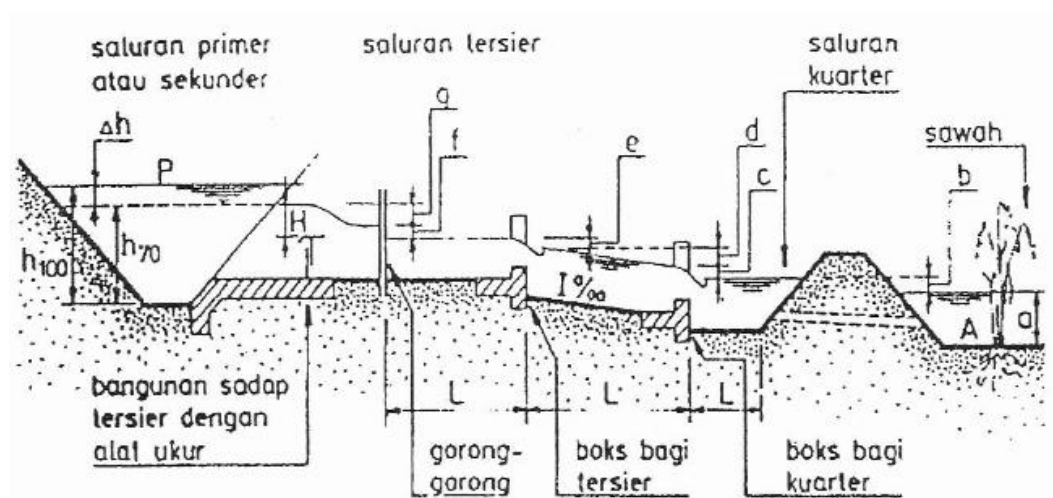
Gambar 2.8 Elevasi Muka Air Di Saluran Primer/Sekunder
