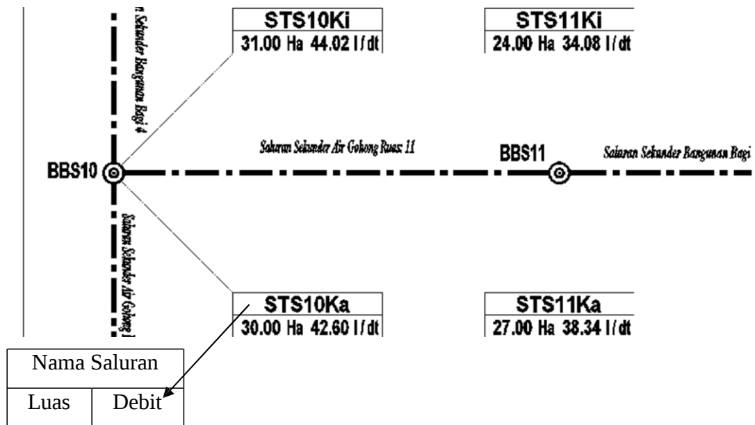
Gambar 2.1 Sket Jaringan Irigasi
