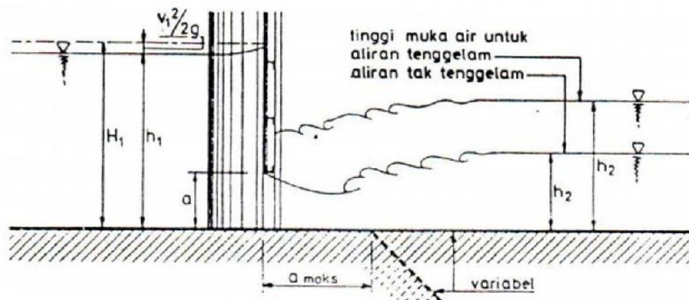
Gambar 2.6 Aliran di Bawah Pintu Sorong dengan Dasar Horizontal
