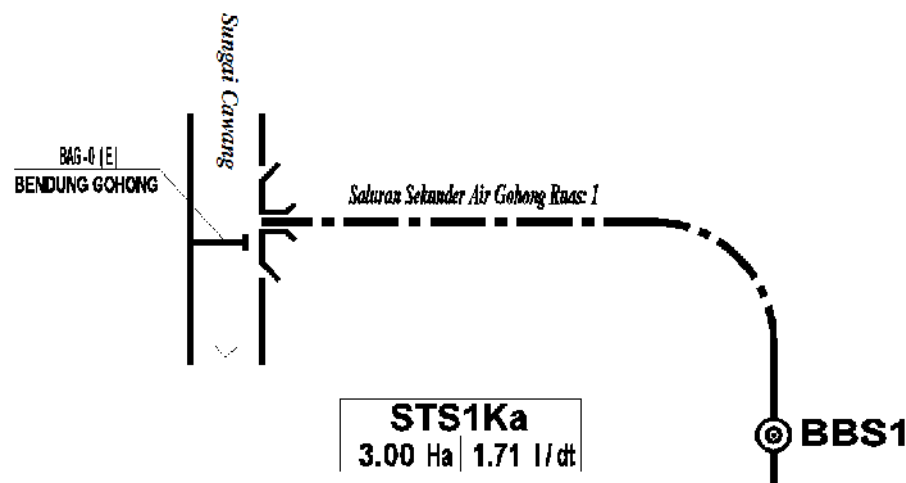
Gambar 2.2 Sket Saluran Sekunder
