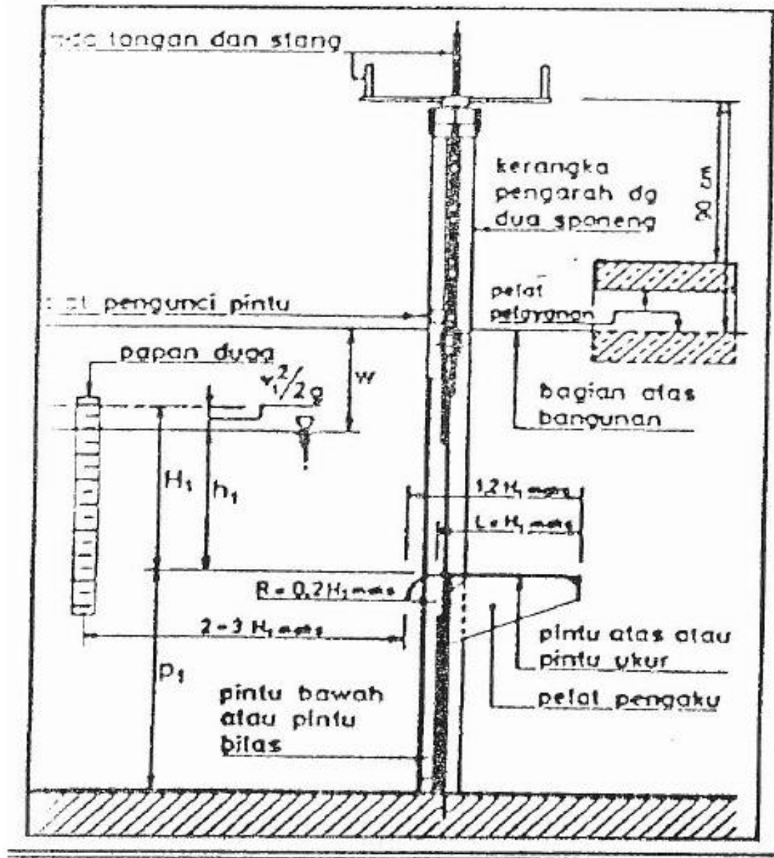
Gambar 2.4 Dimensi Alat Ukur Romiyn dengan Pintu Bawah
