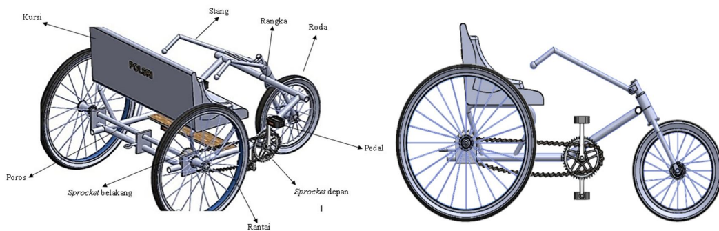
Gambar 2.5 Rancangan Sepeda Gerobak
