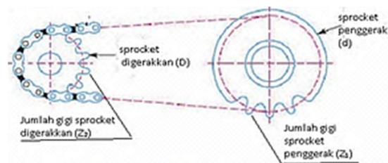
Gambar 2.6 Rantai dan Sprocket
