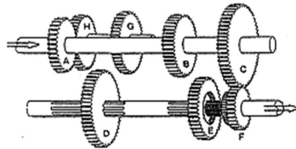
Gambar 2.9 Poros Transmisi Sumber: (9)
