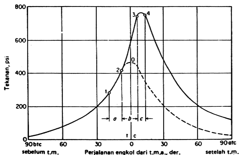
Gambar 2.8 Tingkat pembakaran dalam sebuah mesin (Maleev.V.L, 1995)
