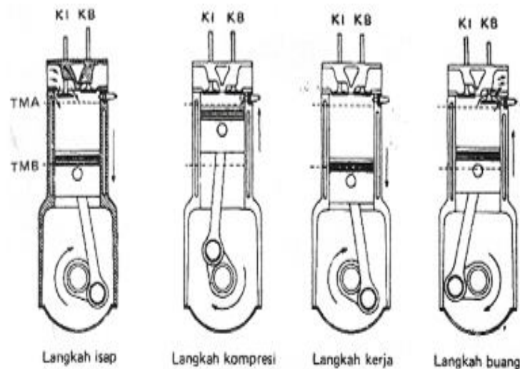
Gambar 2.5 Skema Gerakan Torak 4 langkah (Arismunandar, 2002)
