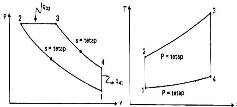
Gambar 2.3 Diagram P-V dan T-S siklus otto (Cengel & Boles, 1994:458)
