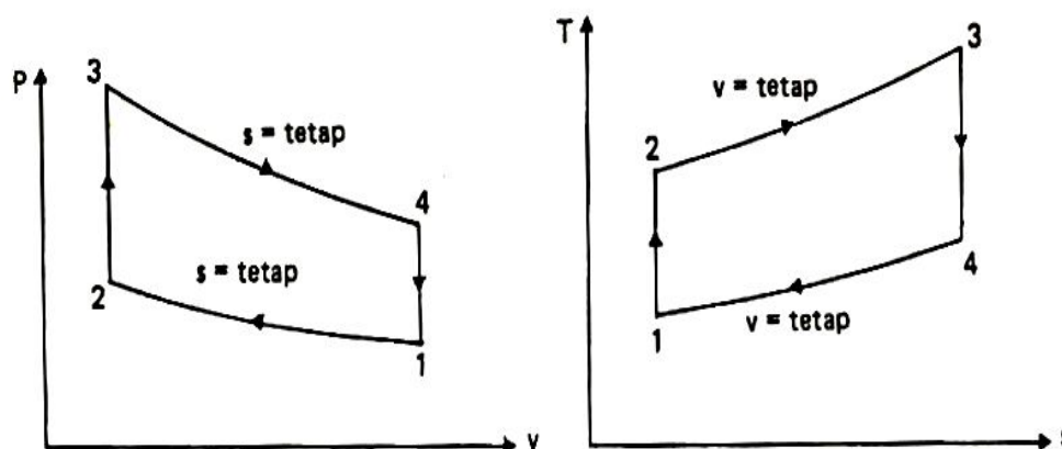
Gambar 2.2 Diagram P-V dan T-S siklus otto (Cengel & Boles, 1994:451)
