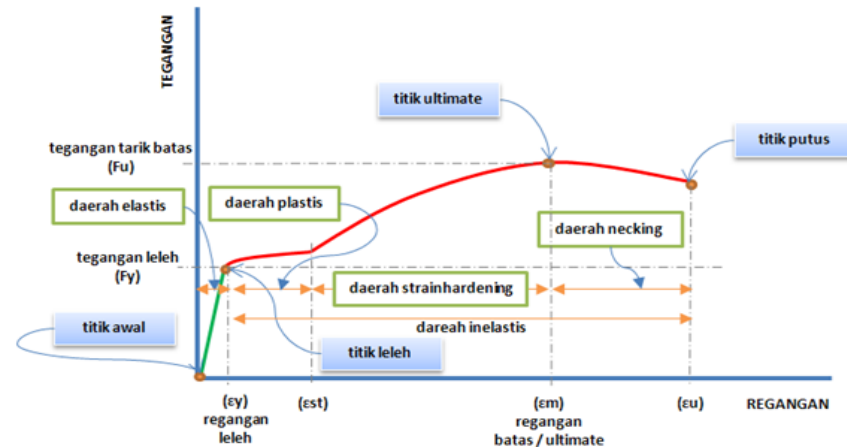
Gambar 2.3 Grafik karbon pada baja tulangan beton (Lit 5 dunduh 27 april 2014)
