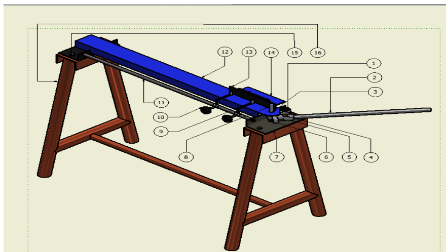
Gambar 2.5 Konstruksi alat manual penekuk begel segiempat
