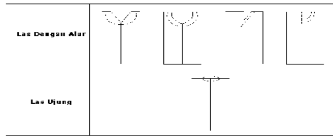
Gambar. 5 Sambungan Sisi
