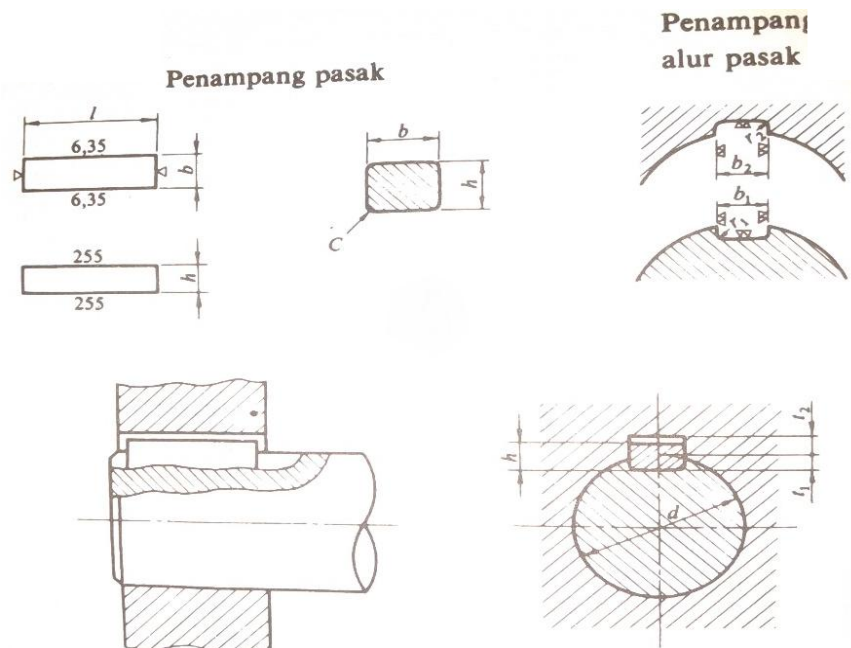
Gambar 2.14. Dimensi pasak
