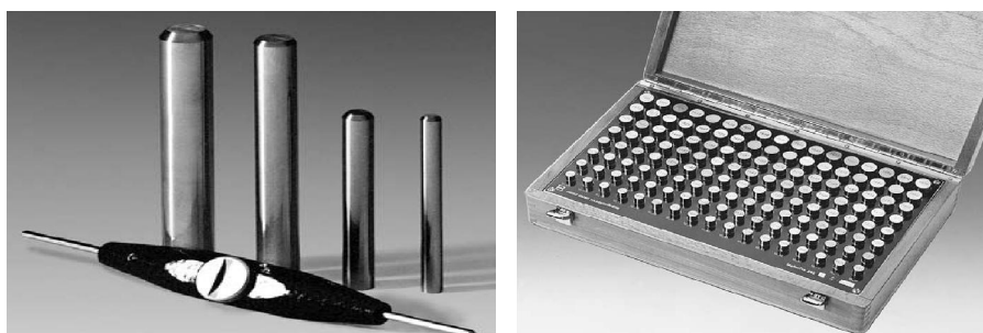
Gambar 2.16 Pin Penepat
