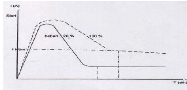
Gambar 2.10 Karakteristik Start Motor Induksi
