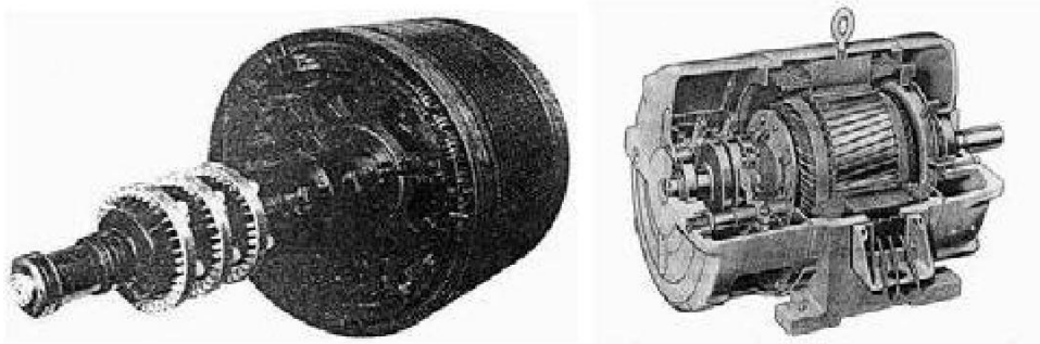
Gambar 2.4 Motor Induksi Rotor Belitan
