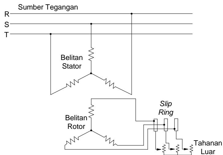
Gambar 2.5 Rangkaian Rotor Lilit
