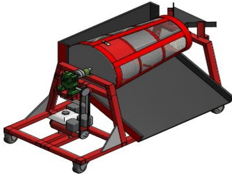
Gambar 2.2 mesin pengayak pasir
