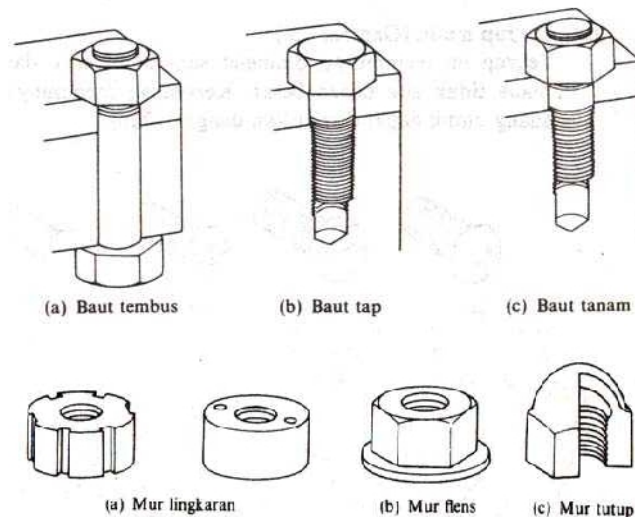
Gambar 2.3.7 Jenis Baut dan Mur
