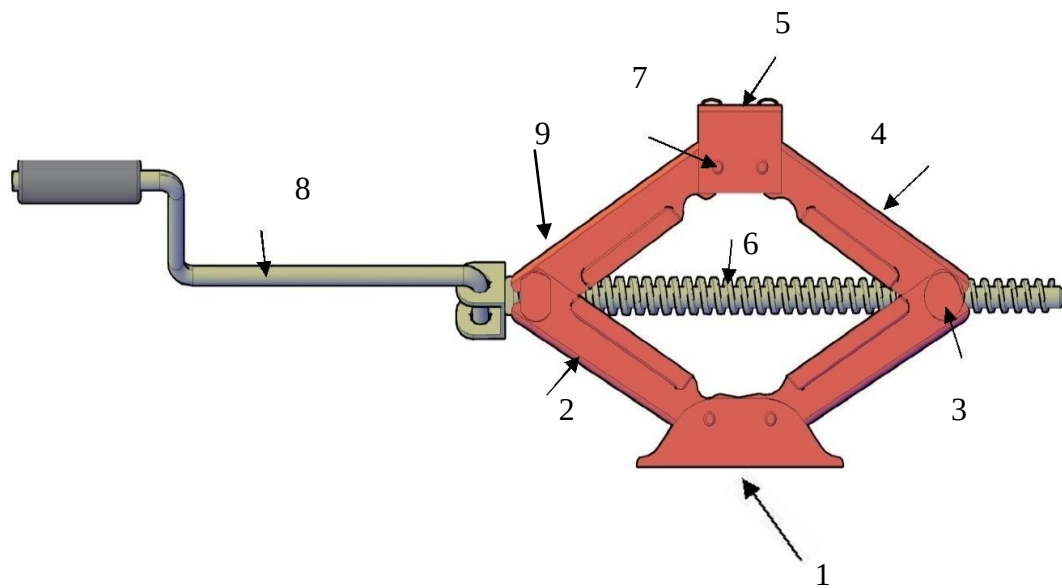
Gambar 2.1 : Komponen-komponen dongkrak ulir mekanis
