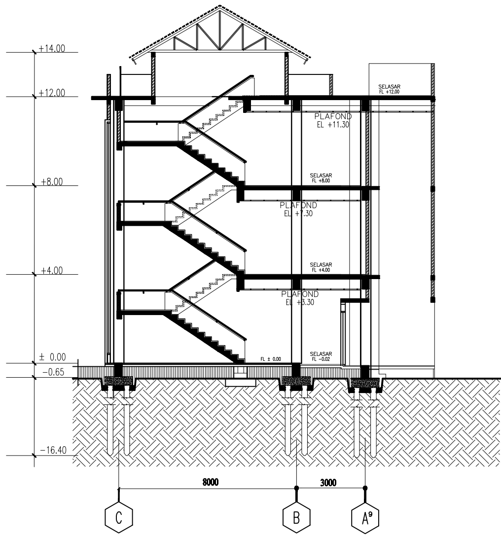
POTONGAN 2 - 2 GEDUNG TEORI SKALA 1:100
