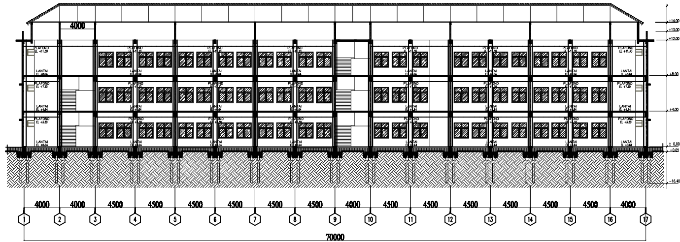
POTONGAN 1-1 GEDUNG TEORI SKALA 1:250
