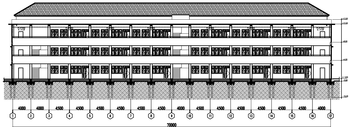
POTONGAN 3-3 GEDUNG TEORI SKALA 1:250
