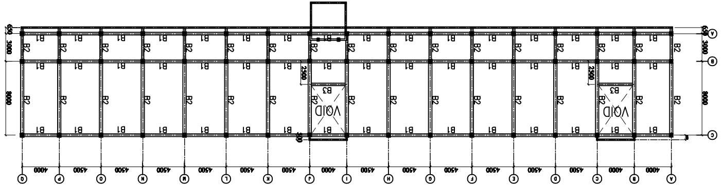
DENS BALOK LANTAI 2 SKALA 1 : 250
