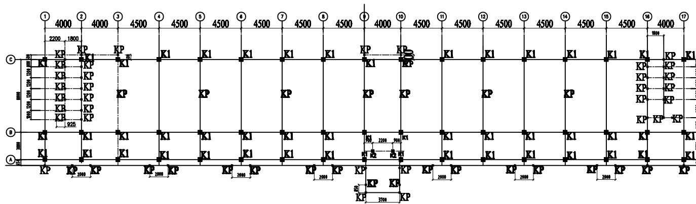
DENAH KOLOM LANTAI 2 SKALA 1 : 250
