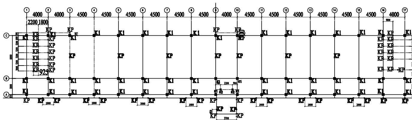
DENAH KOLOM LANTAI 3 SKALA 1 : 250
