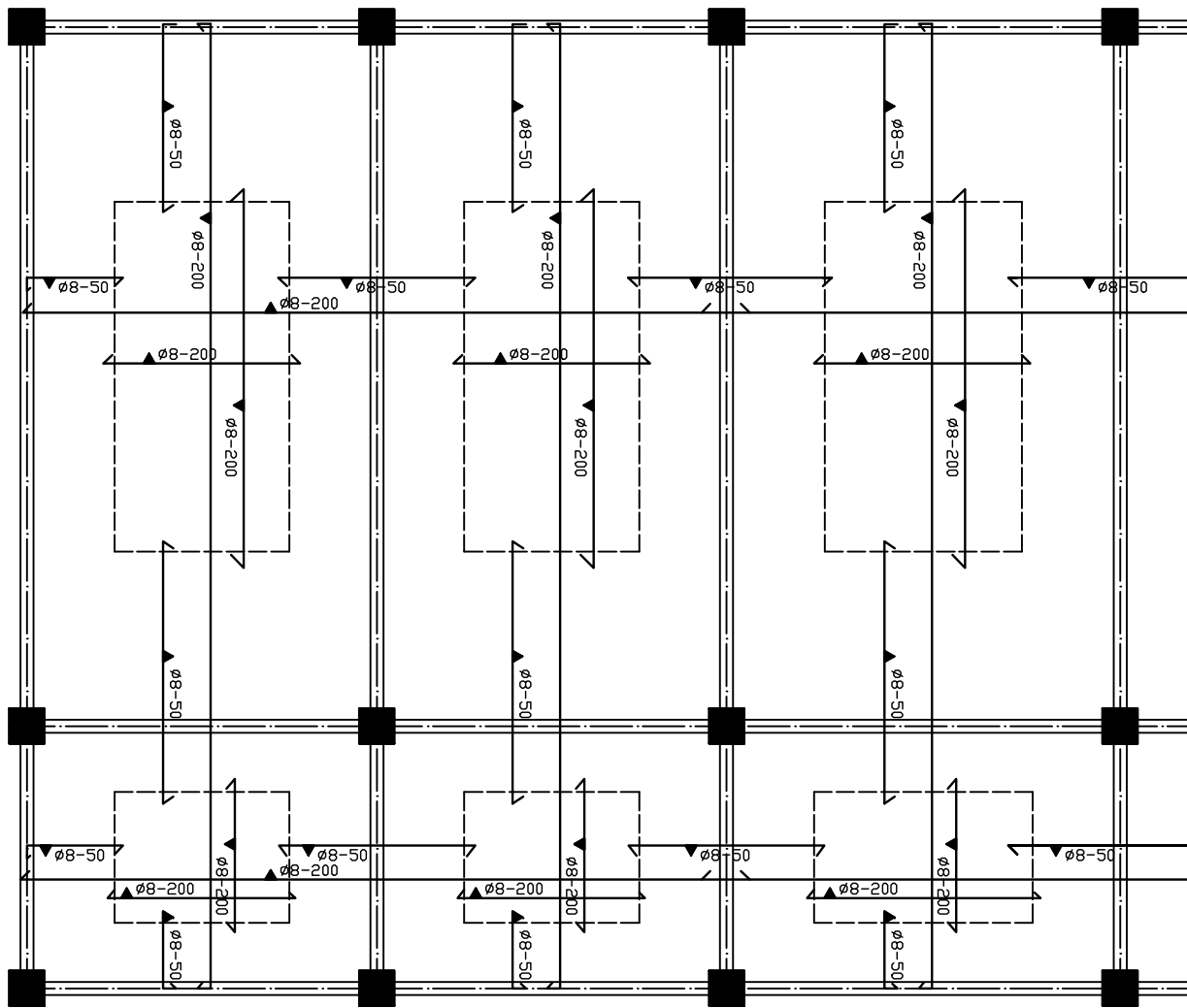
— — DETAIL PELAT LANTAI SKALA 1 : 5
