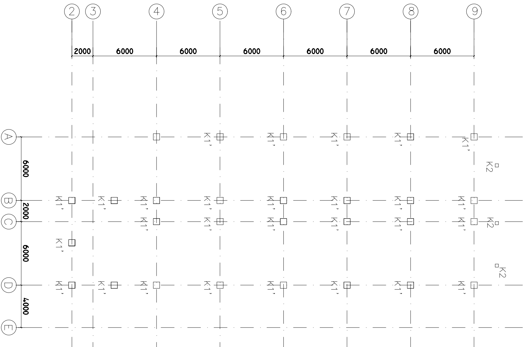
1 DENAH KOLOM LANTAI DUA SKALA 1 : 200
