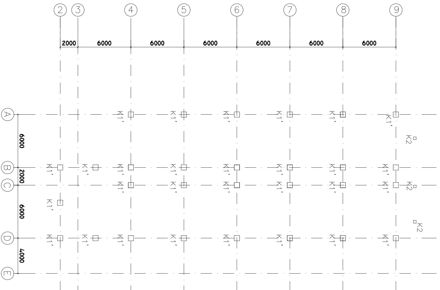
1 DENAH KOLOM LANTAI SATU 008 008 SKALA 1 : 200
