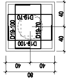
DETAIL P-2 ( 12 UNIT ) Skala 1 : 25
