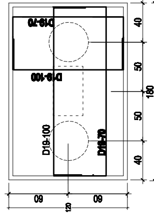
DETAIL P-1 ( 24 UNIT ) Skala 1 : 25
