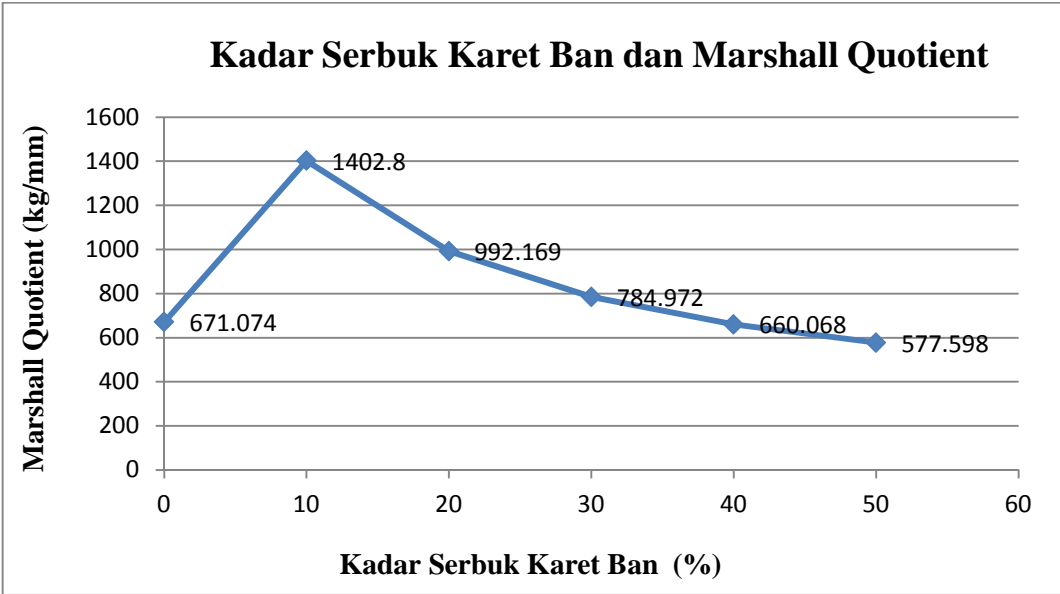
Grafik Hubungan Penambahan Kadar Serbuk Karet Ban dan Marshall Quotient
