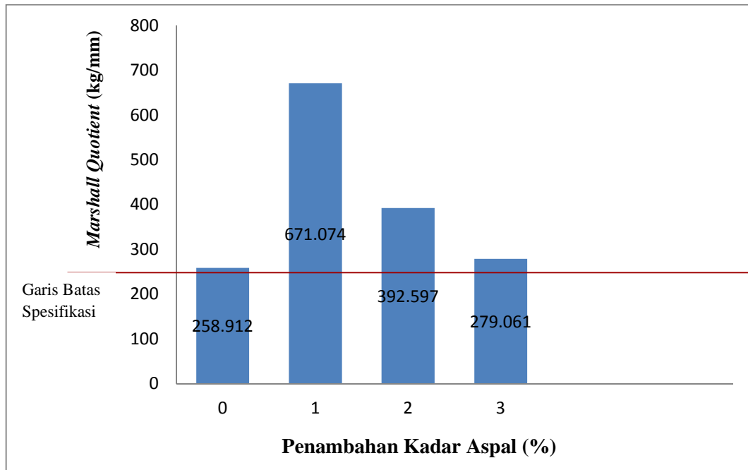
Grafik Histogram Marshall Quotient Campuran Daur ulang Dengan Penambahan Kadar Aspal
