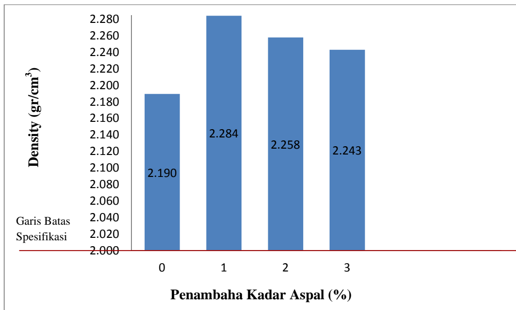
Grafik Histogram Density Campuran Daur Ulang Dengan Penambahan Kadar Aspal
