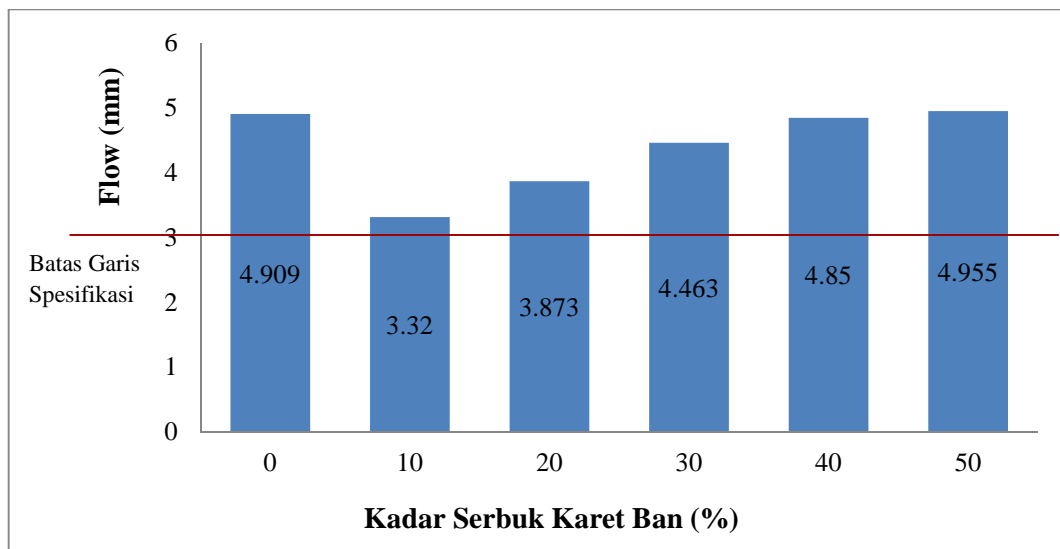
Grafik Histogram Flow Campuran Daur Ulang Dengan Penambahan Serbuk Karet Ban
