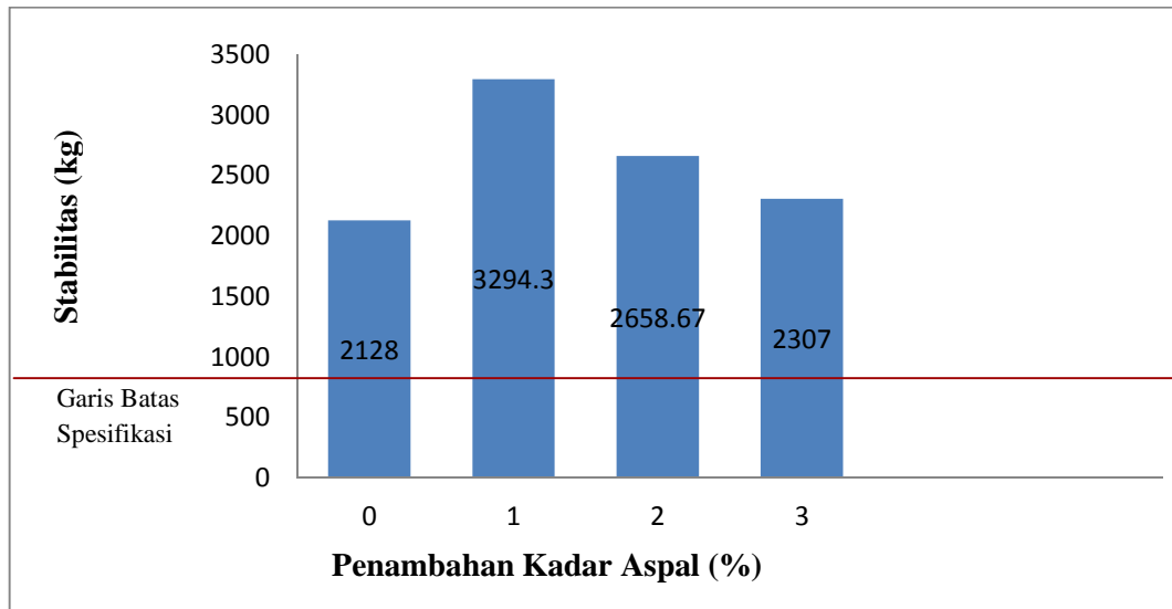
Grafik Histogram Stabilitas Campuran Daur Ulang Dengan Penambahan Kadar Aspal
