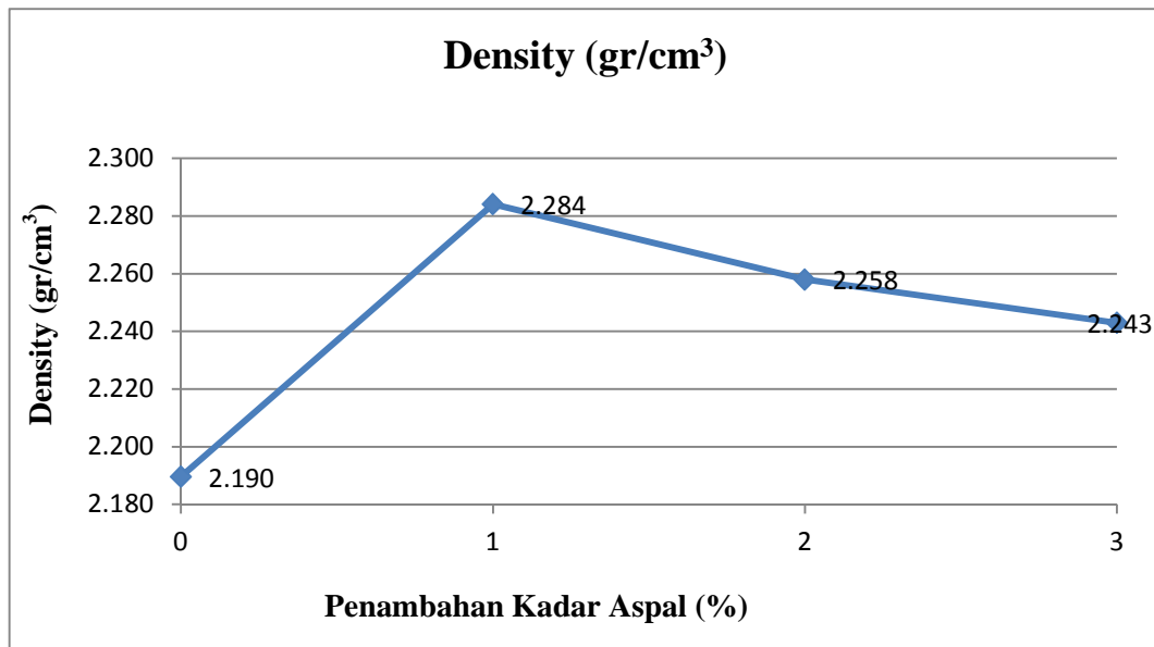
Grafik Hubungan Penambahan Kadar Aspal dan Density
