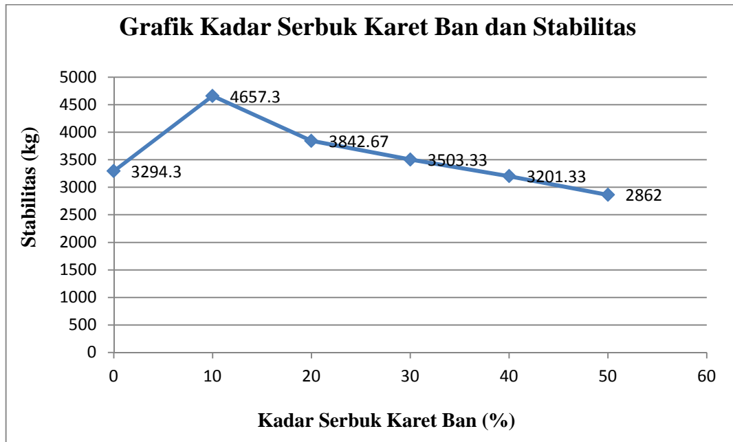
Grafik Hubungan Penambahan Kadar Serbuk Karet Ban dan Stabilitas
