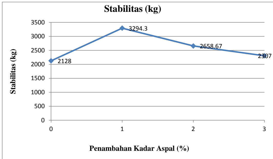
Grafik Hubungan Penambahan Kadar Aspal dan Stabilitas
