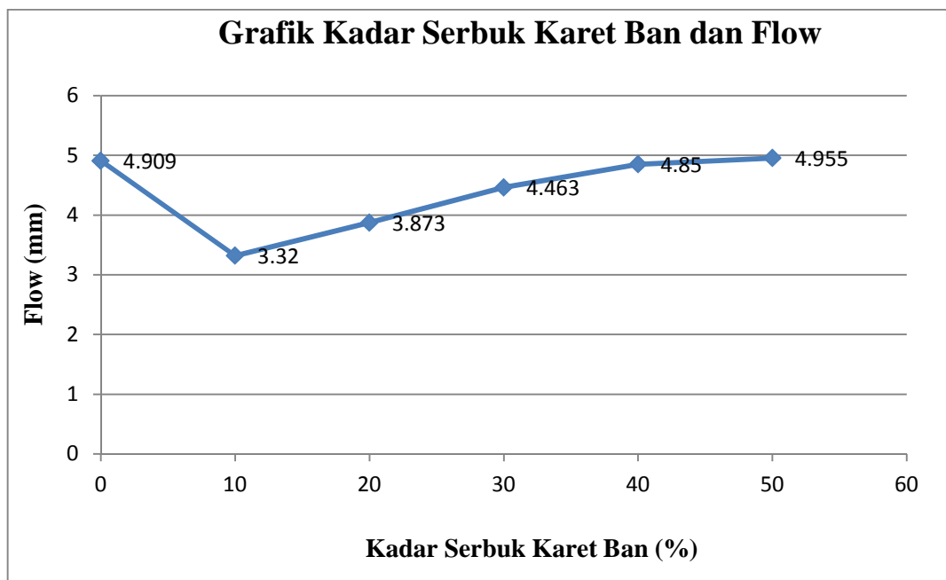
Grafik Hubungan Penambahan Kadar Serbuk Karet Ban dan Flow
