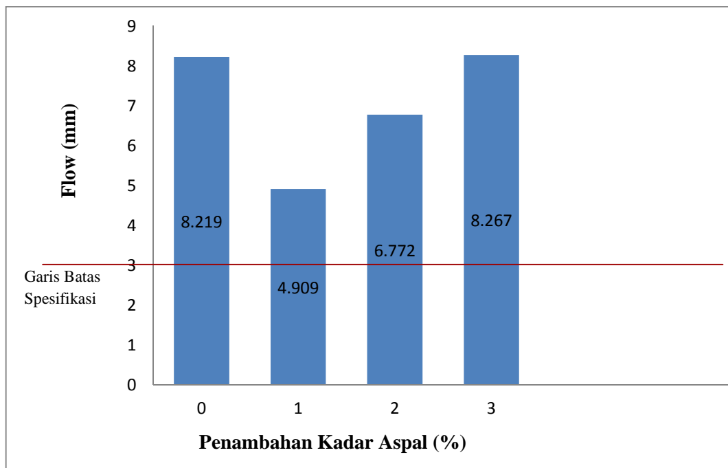
Grafik Histogram Flow Campuran Daur Ulang Dengan Penambahan Kadar Aspal
