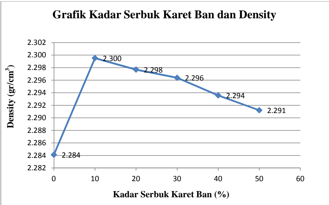
Grafik Hubungan Penambahan Kadar Serbuk Karet Ban dan Density
