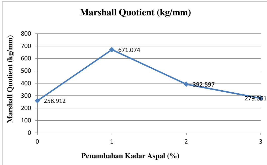
Grafik Hubungan Penambahan Kadar Aspal dan Marshall Quotient
