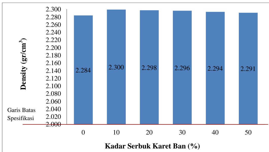
Grafik 4.16 Histogram Density Campuran Daur Ulang Dengan Penambahan Serbuk Karet Ban
