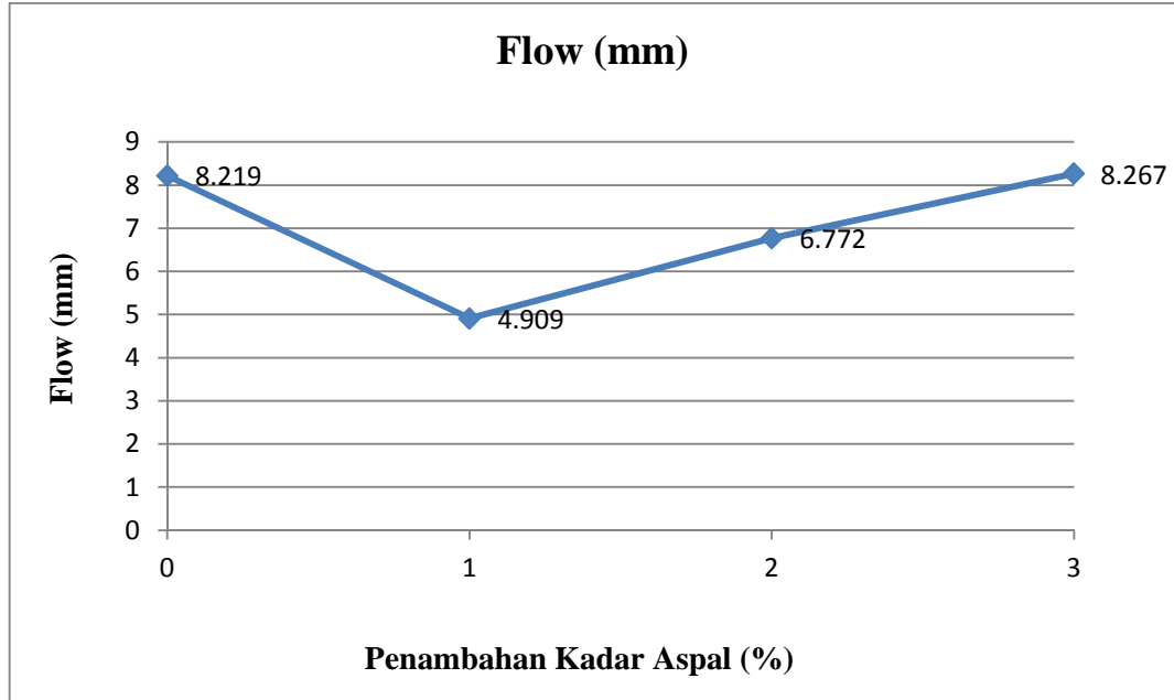
Grafik Hubungan Penambahan Kadar Aspal dan Flow
