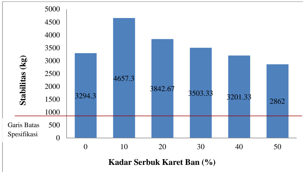
Grafik Histogram Stabilitas Campuran Daur Ulang Dengan Penambahan Serbuk Karet Ban
