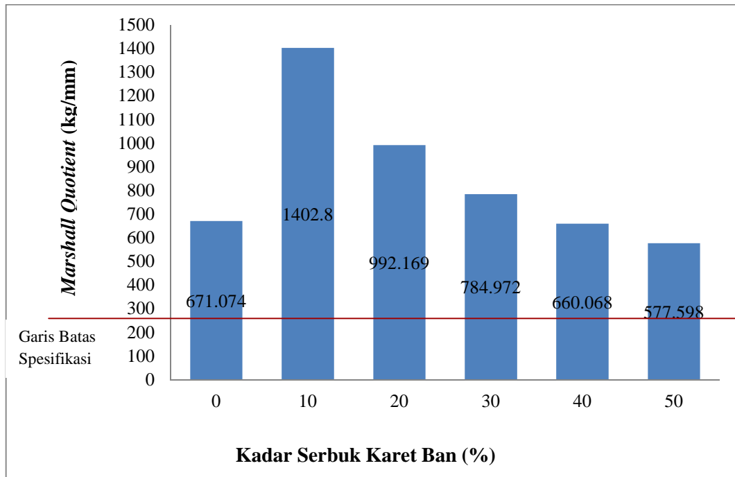
Grafik Histogram Marshall Quotient Campuran Daur Ulang Dengan Penambahan Serbuk Karet Ban
