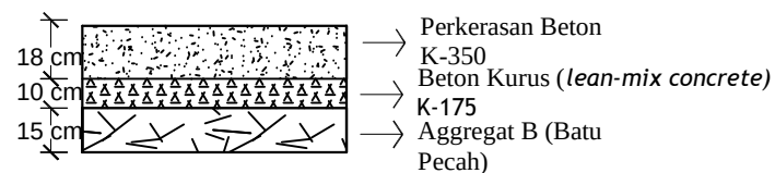
POTONGAN 1-1 SKALA 1:20
