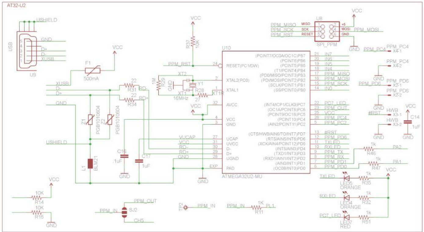
Rangkaian AT32-U2
