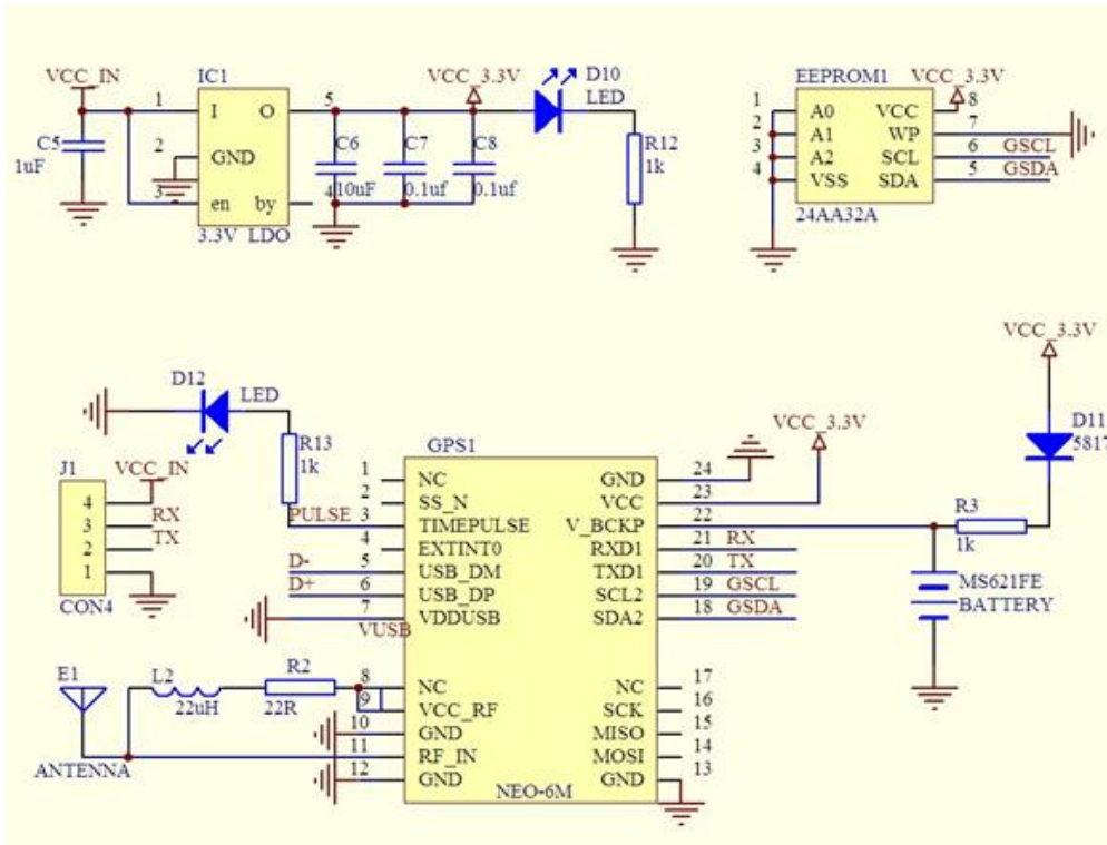
Gambar Rangkaian GPS
