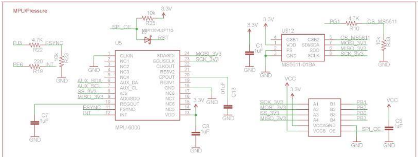
Rangkaian MPU (Gyroscope dan Accelerometer)
