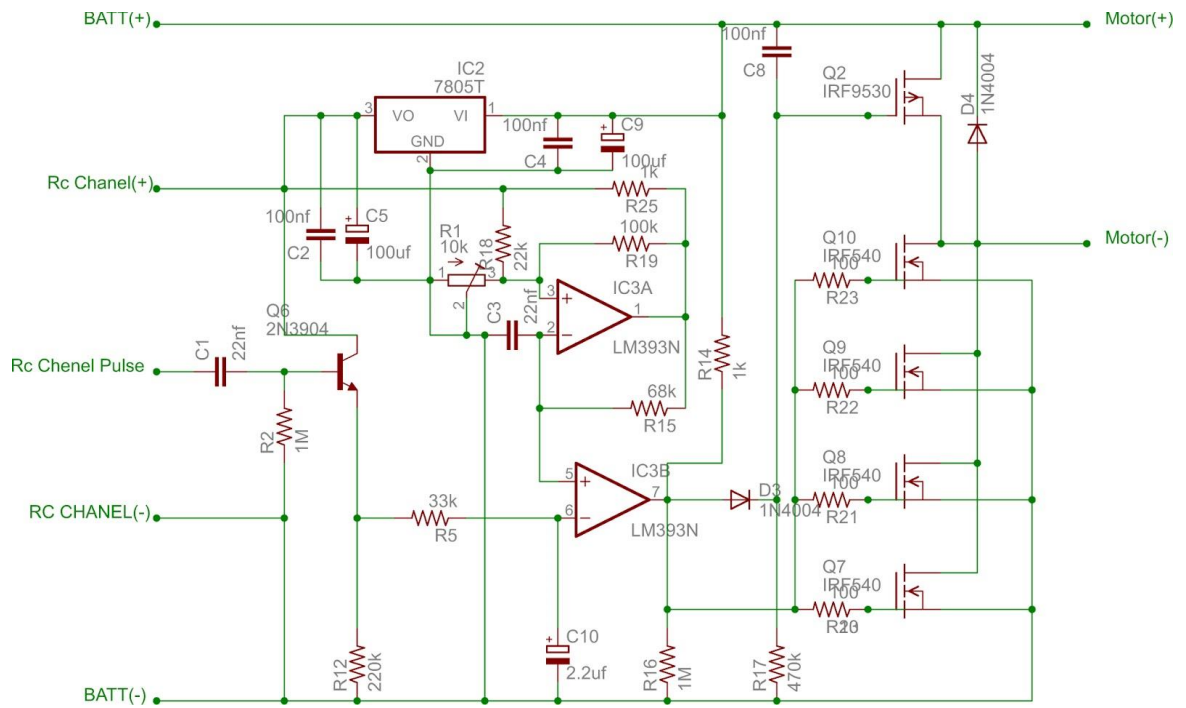
Rangkaian ESC
