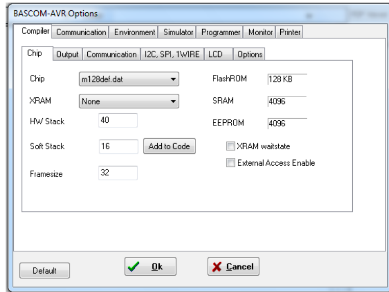
Gambar 2.10 Jendela Option
