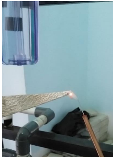
Gambar 23. Uji Bakar terhadap Alumunium
