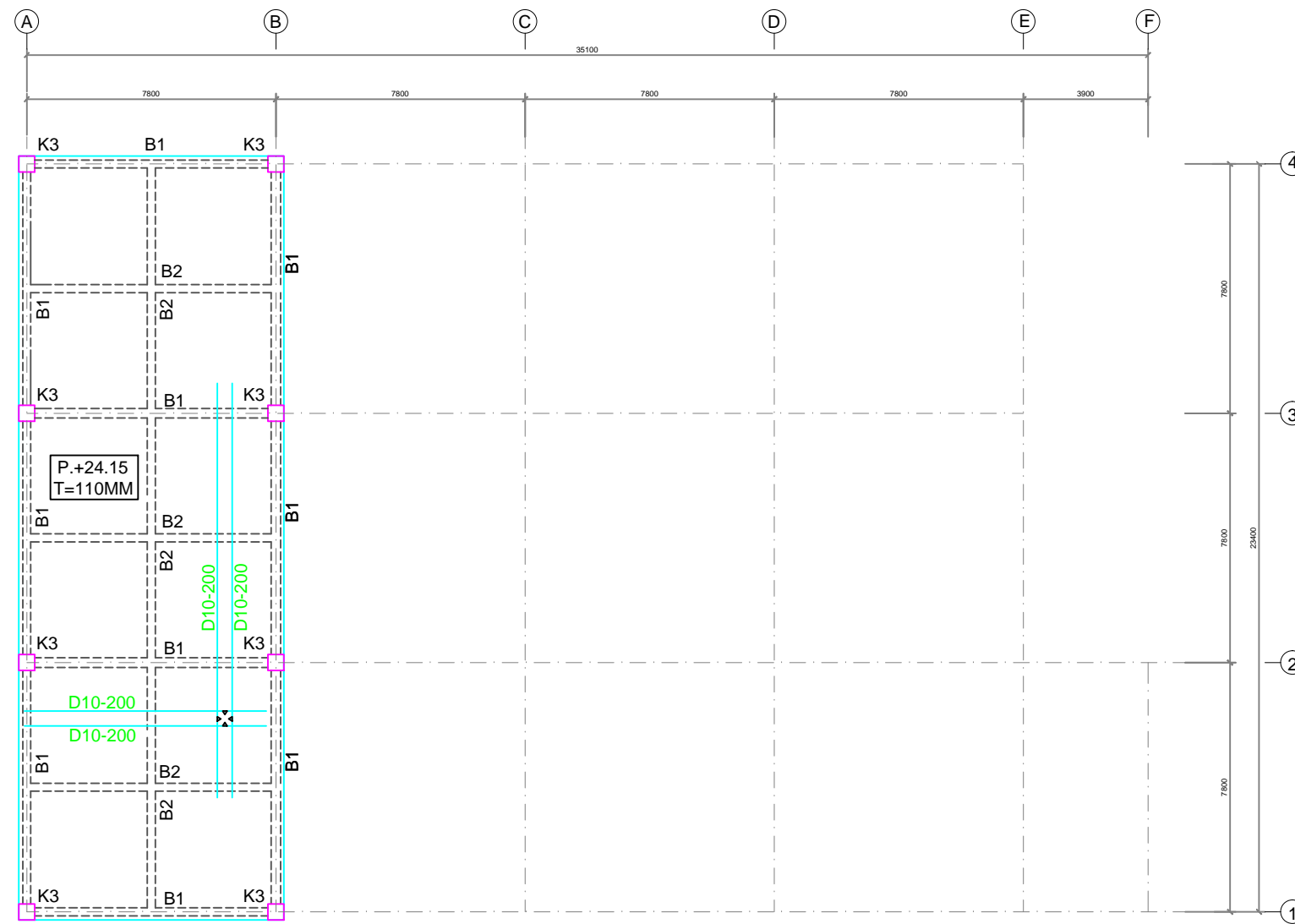
DENAH PEMBALOK LANTAI DAK ATAP SKALA 1 : 100
