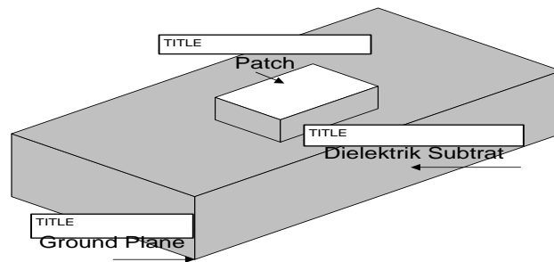
Gambar 1. Struktur Antena Mikrostrip
