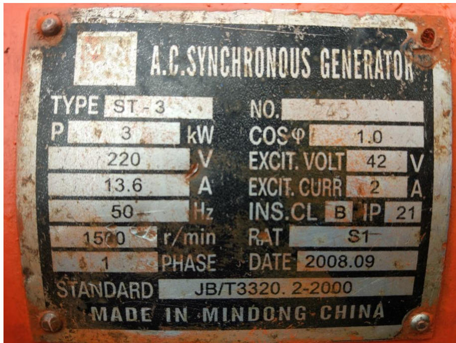
Nameplate Generator Sinkron Satu Fasa
