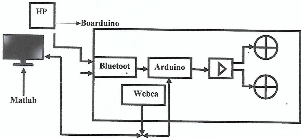
Blok Diagram Rancang Bangun Robot Kontrol Digital dan Monitoring Menggunakan Matlab
