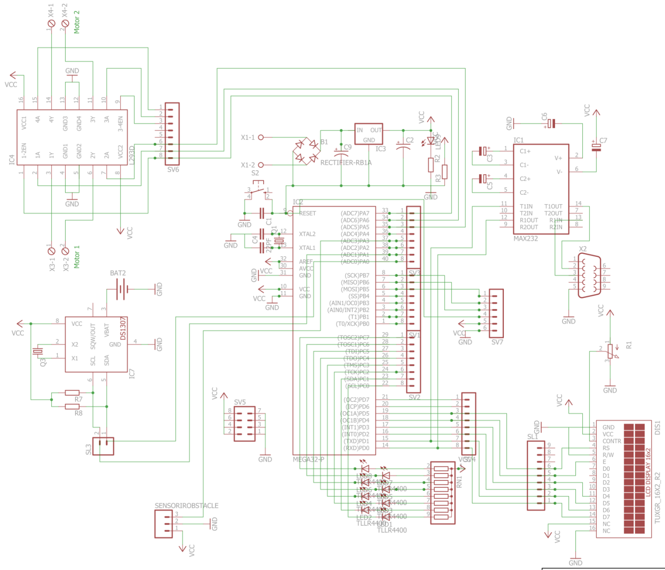
Gambar 3.8 Skematik Rangkaian Keseluruhan
