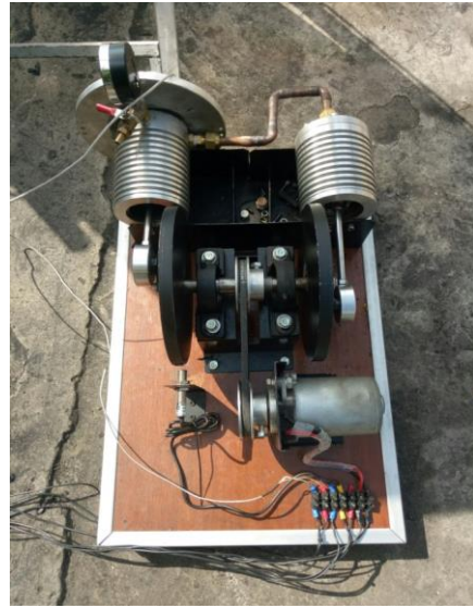
Mesin Stirling
