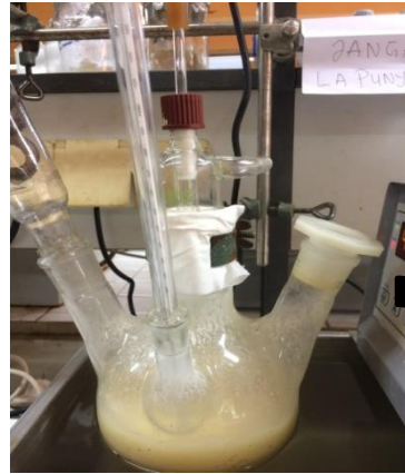
Proses Sulfonasi
