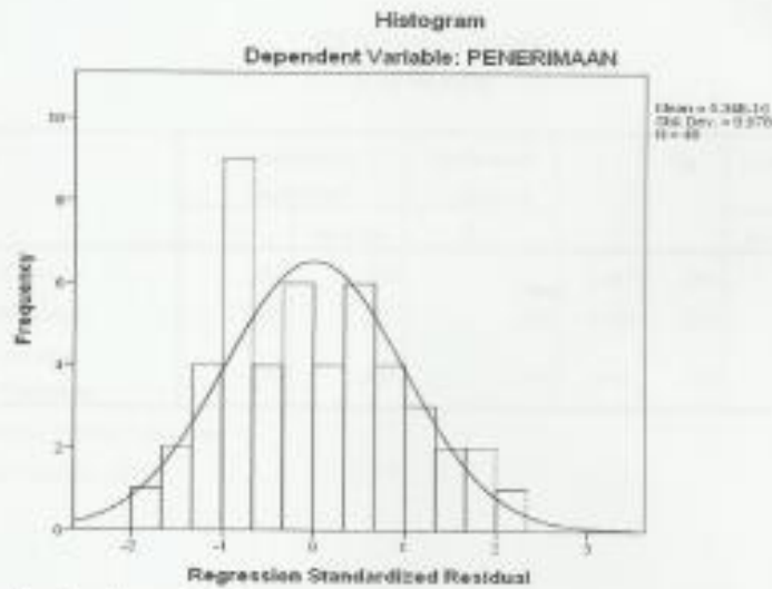
Gambar 4.2 Grafik Histogram
