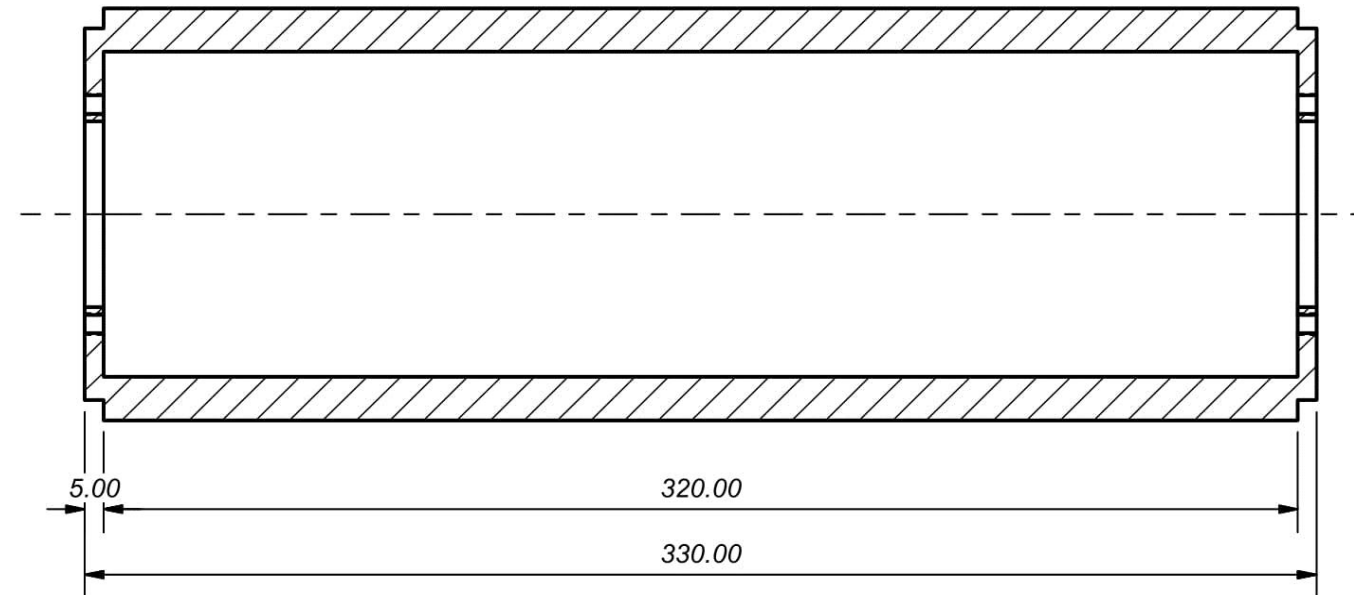
SECTION G-G SCALE 1 : 2
