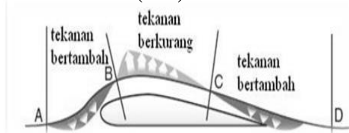
Gambar 2.14 Tekanan pada airfoil
