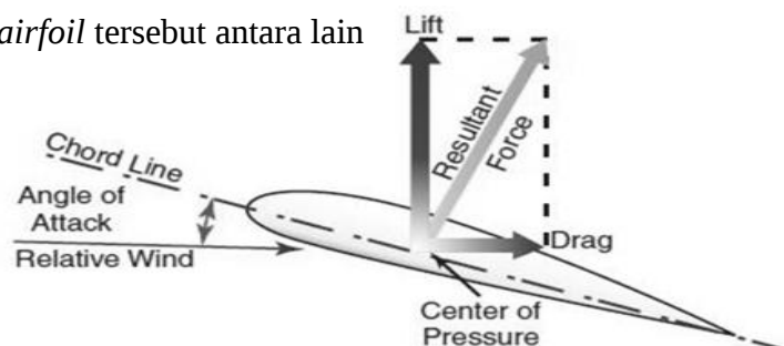
Gambar 2.16 Gaya pada airfoil
