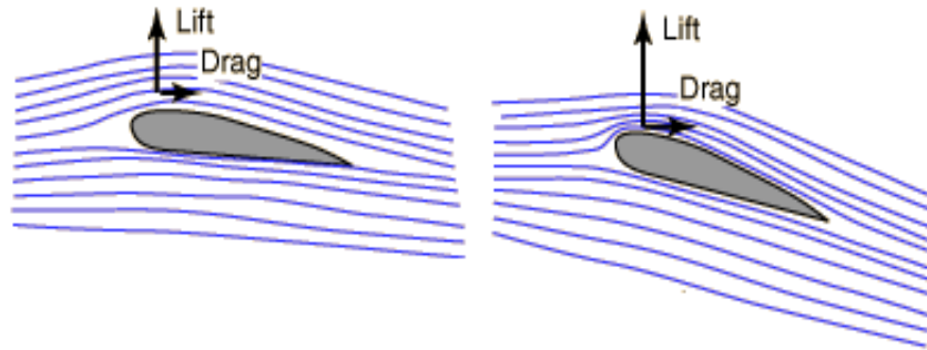
Gambar 2.9 Aliran laminar
