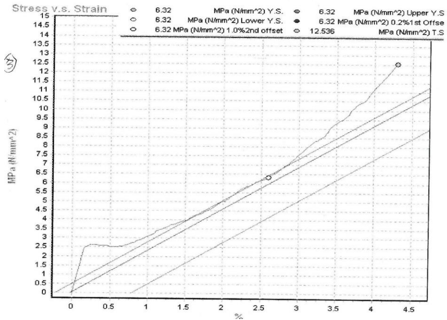
Grafik Uji Tarik 2 Lapisan Serat Acak Vakum
