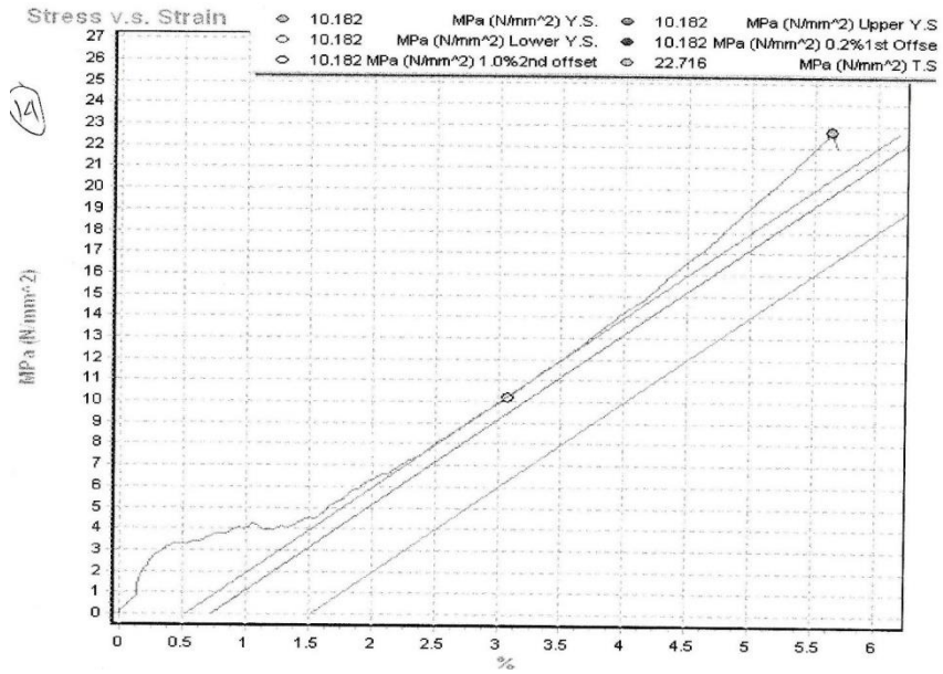
Grafik Uji Tarik 2 Lapisan Serat Melintang Vakum
