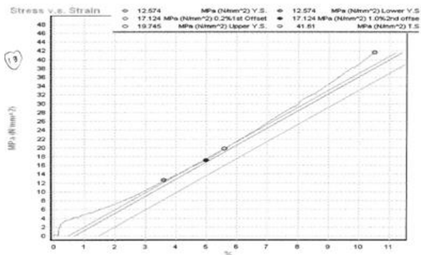
Grafik Uji Tarik 1 Lapisan Serat Lurus Vakum
