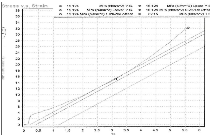
Grafik Uji Tarik 2 Lapisan Fiberglass Tekan
