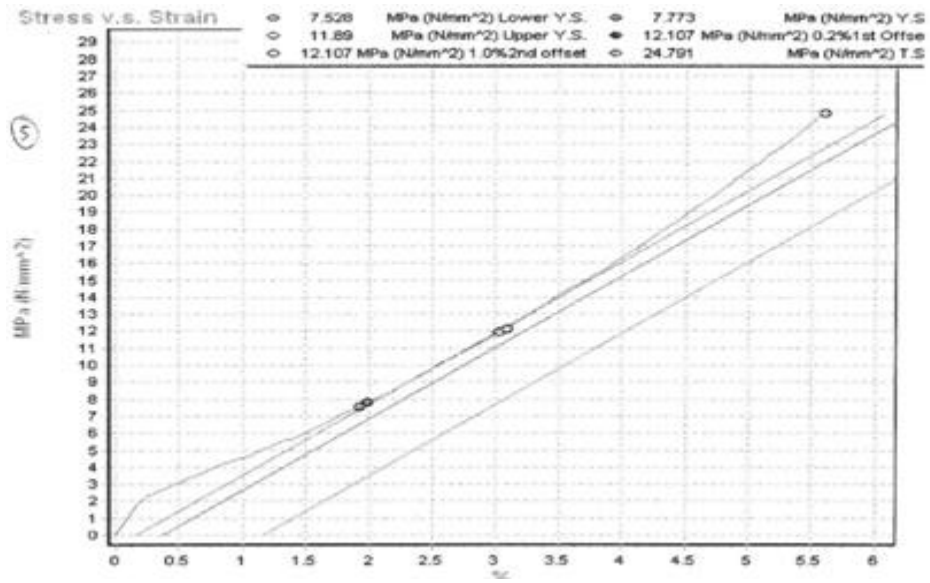
Grafik Uji Tarik 1 Lapisan Serat Acak Tekan
