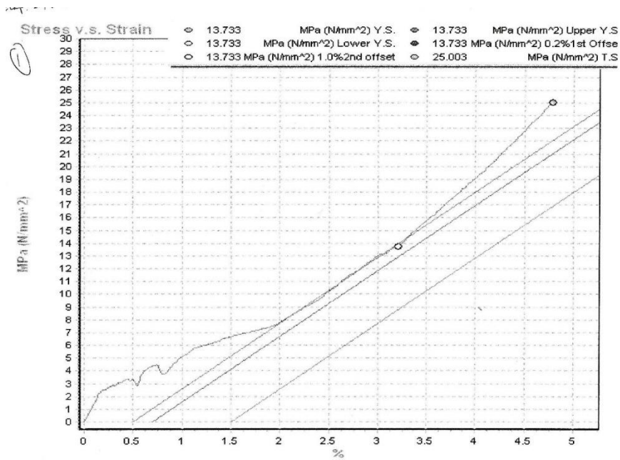
Grafik Uji Tarik 2 Lapisan Serat Lurus Vakum
