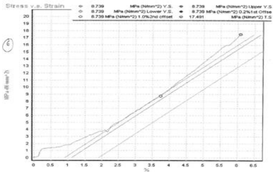
Grafik Uji Tarik 1 Lapisan Serat Melintang Vakum
