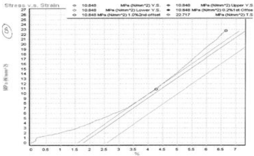
Grafik Uji Tarik 1 Lapisan Serat Melintang Tekan
