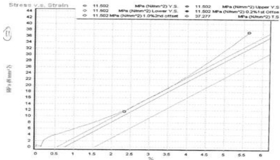
Grafik Uji Tarik 1 Lapisan Fiberglass Vakum
