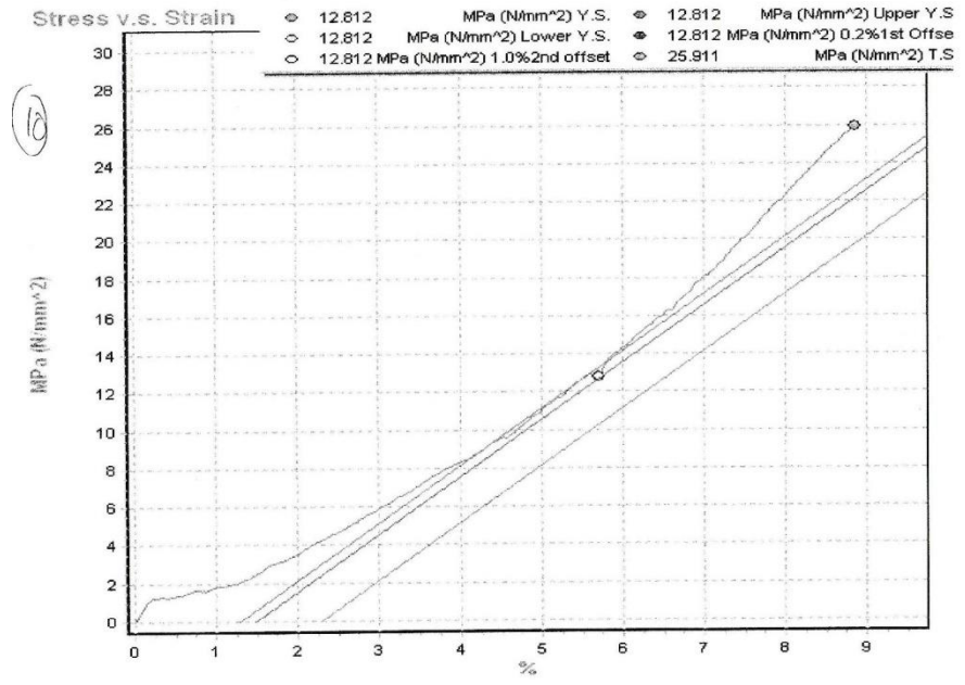
Grafik Uji Tarik 2 Lapisan Serat Acak Tekan
