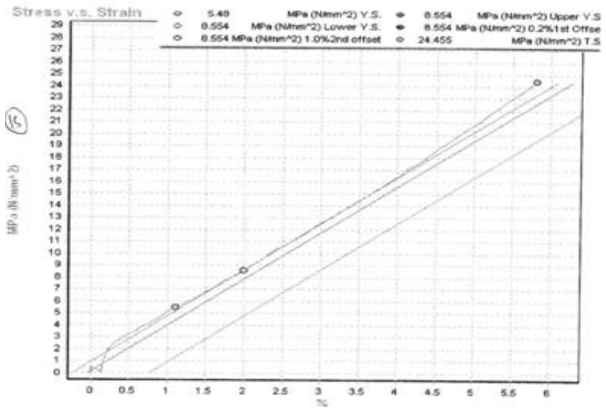
Grafik Uji Tarik 1 Lapisan Fiberglass Tekan
