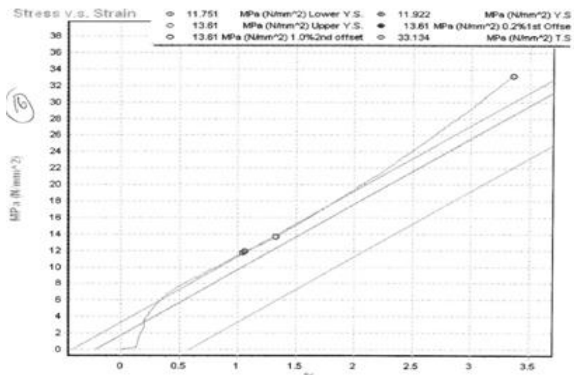
Grafik Uji Tarik 1 Lapisan Serat Acak Vakum
