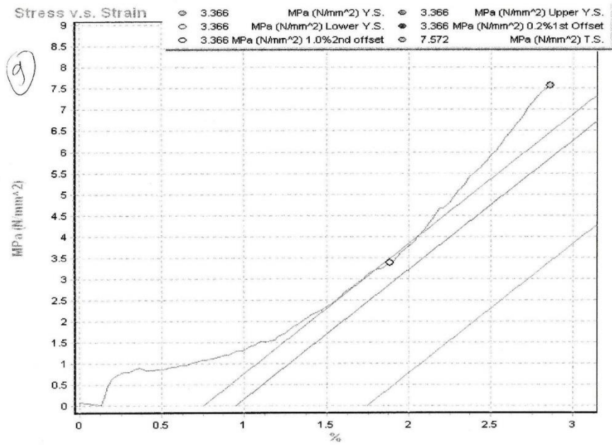
Grafik Uji Tarik 2 Lapisan Serat Lurus Tekan
