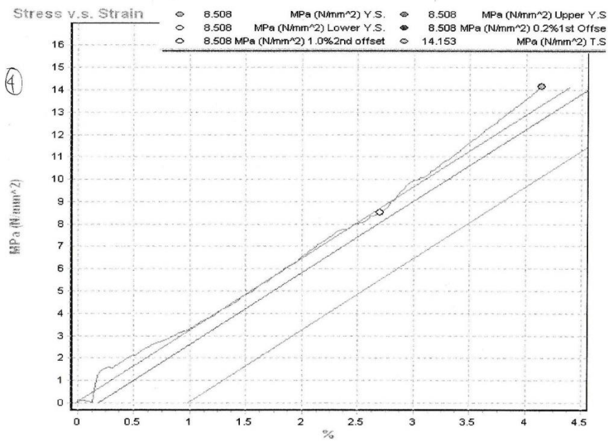
Grafik Uji Tarik 2 Lapisan Serat Melintang Tekan
