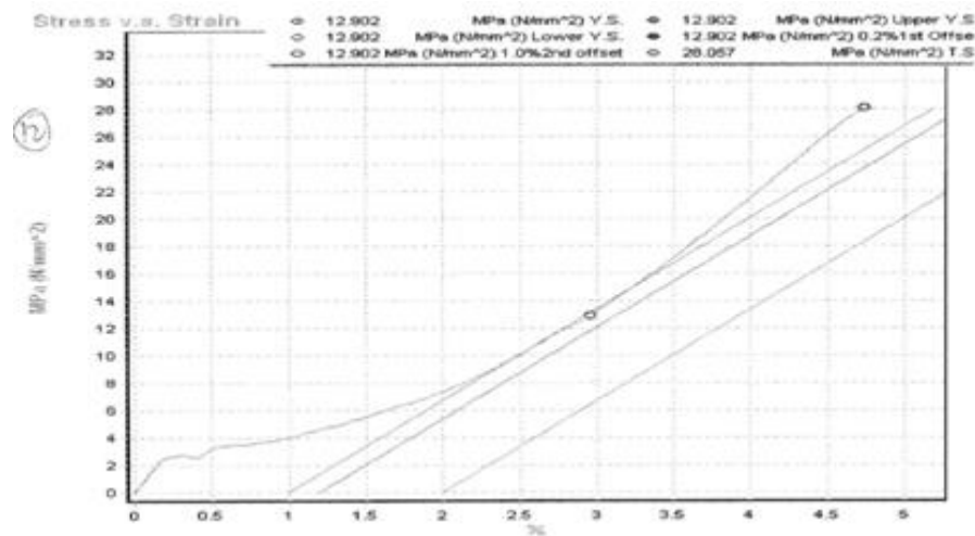
Grafik Uji Tarik 1 Lapisan Serat Lurus Tekan
