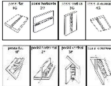
Gambar 2.3 Posisi Pengelasan
