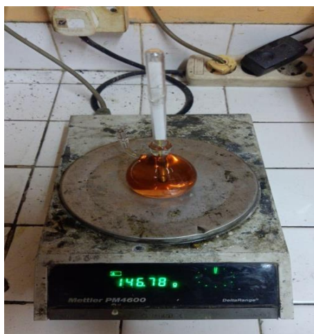
Gambar C.20. Analisa Densitas dan Viskositas Biodisel
