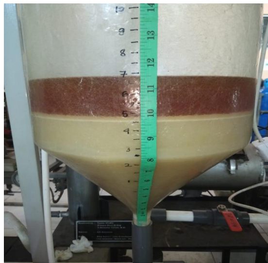
Gambar C.16. Proses Pencucian Biodiesel Menggunakan Air dengan Suhu 60°C Sebanyak 5-6 Kali Pencucian dan Memisahnya
