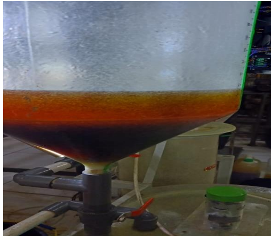
Gambar C.15. Proses Pemisahan Biodiesel dan Gliserol
