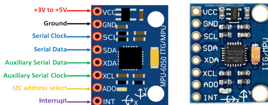
Gambar 2. 5 Modul MPU-6050
